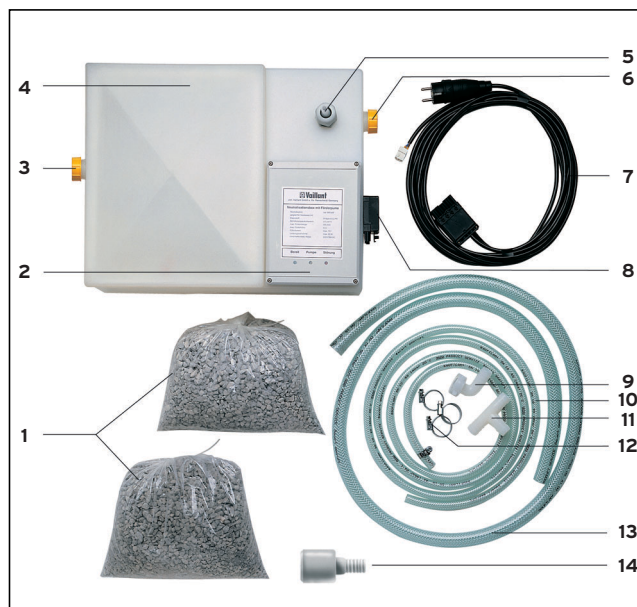
Рис. 1 Подключение устройства нейтрализации с перекачивающим насосом
