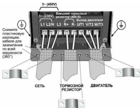
Рисунок 3.5: Подключение силовых кабелей преобразователя Vacon 10, M12 - M13
