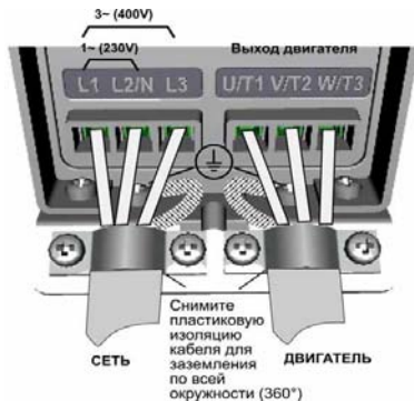
Рисунок 3.4: Подключение силовых кабелей преобразователя Vacon 10, M11
