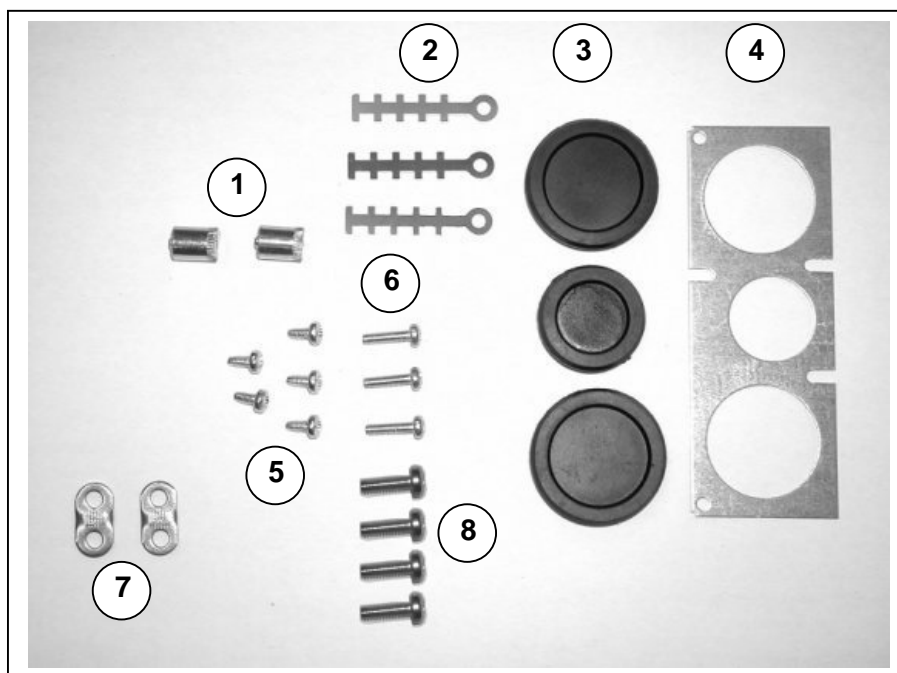
Рис. 6-1. Арматура кабелей
