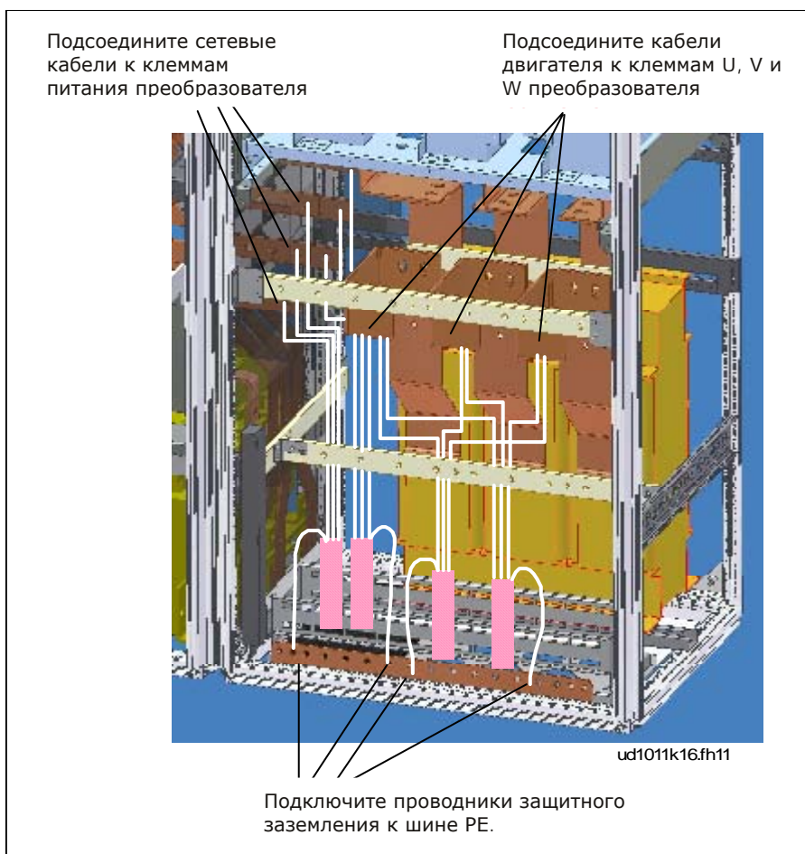
Рисунок 6-5. Разводка силовых кабелей, корпус типоразмера FR14 с подводом кабелей снизу
