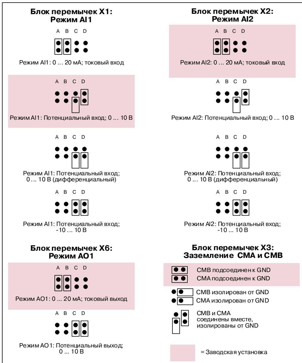
Рисунок 7-9. Выбор переключателей на плате OPT-A1
