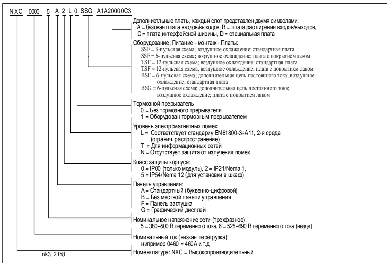
Рисунок 3-1. Код преобразователя частоты Vacon NXC
