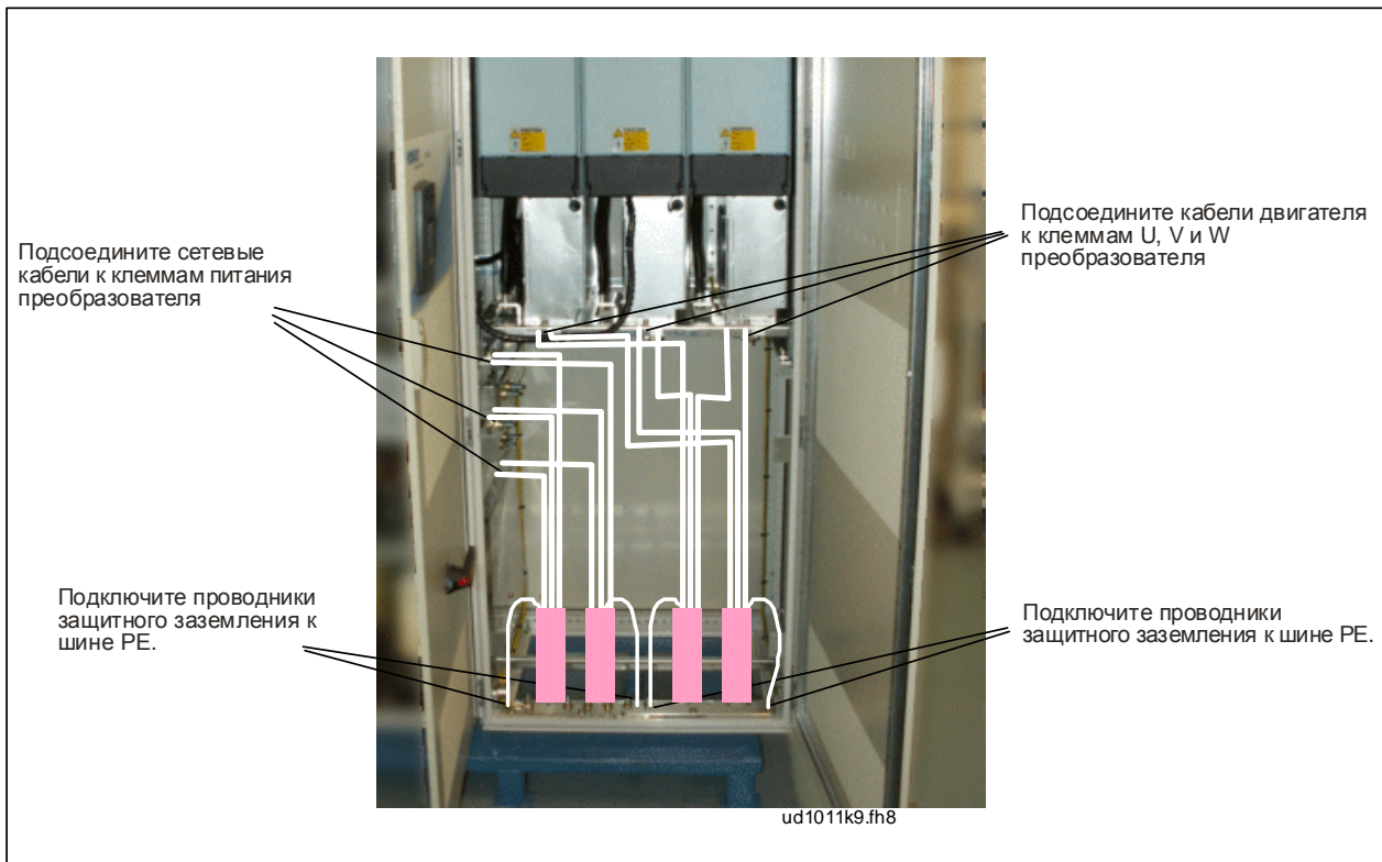
Рисунок 6-4. Прокладка кабелей питания, ввод кабеля снизу для типоразмера FR13
