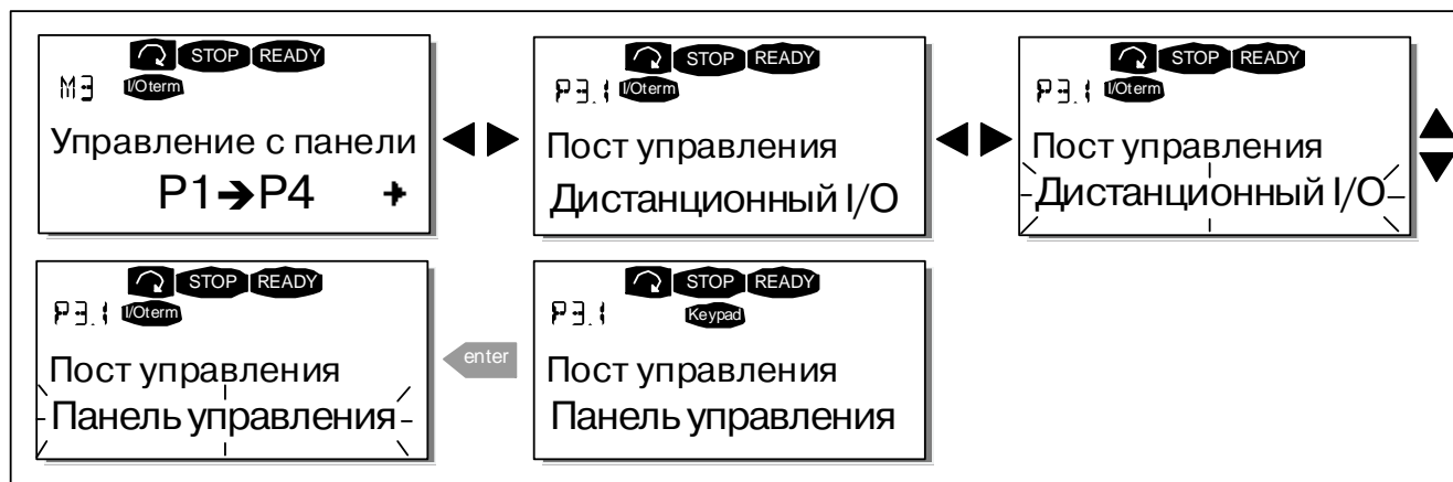
Рисунок 8-6. Выбор поста управления
