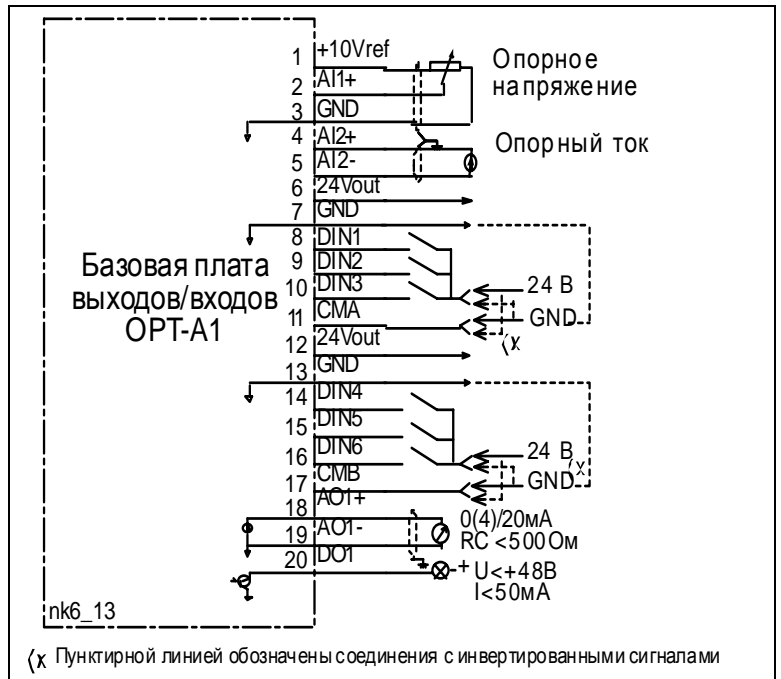
Рисунок 7-4. Принципиальная схема подсоединения базовой платы входов/выходов (OPT-A1)
