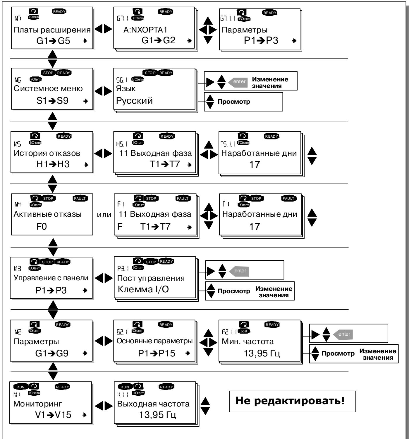
Рисунок 8-3. Схема навигации по меню панели управления
