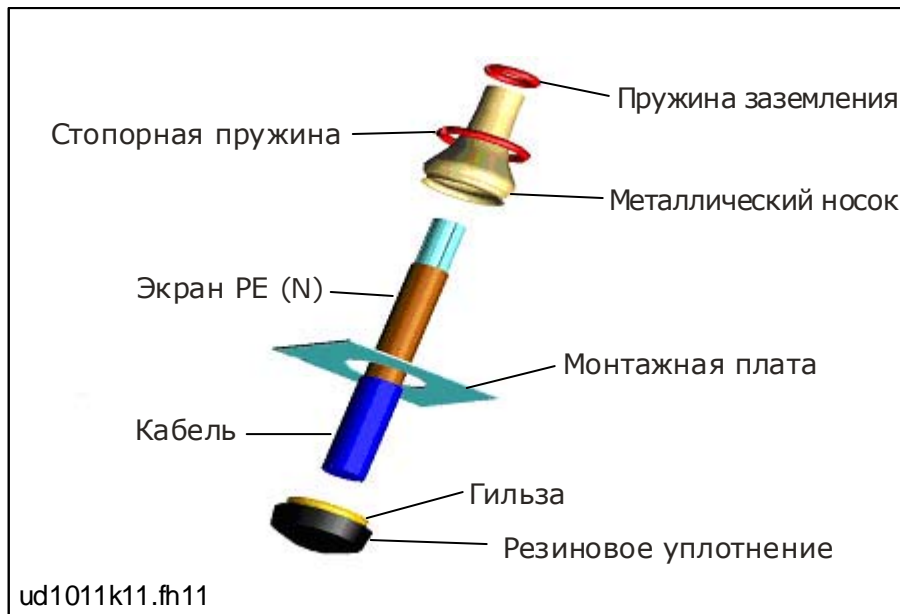
Рисунок 6-7. Детали комплекта кабельного сальника
