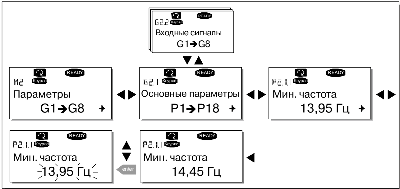
Рисунок 8-5. Процедура изменения параметров
