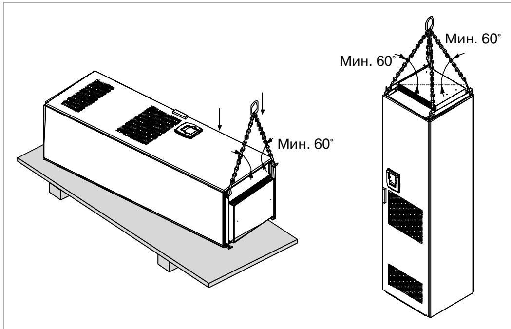
Рисунок 5-2. Подъем устройства
