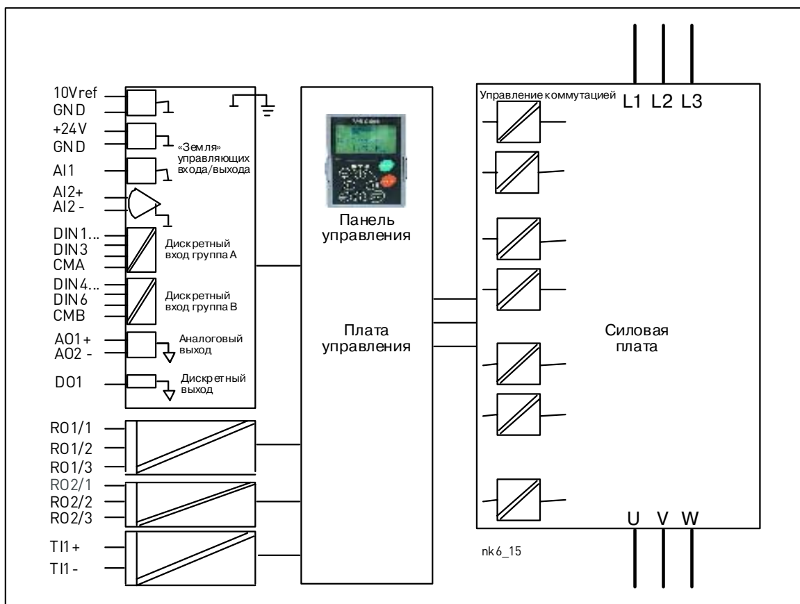
Рисунок 7-6. Гальваническая развязка
