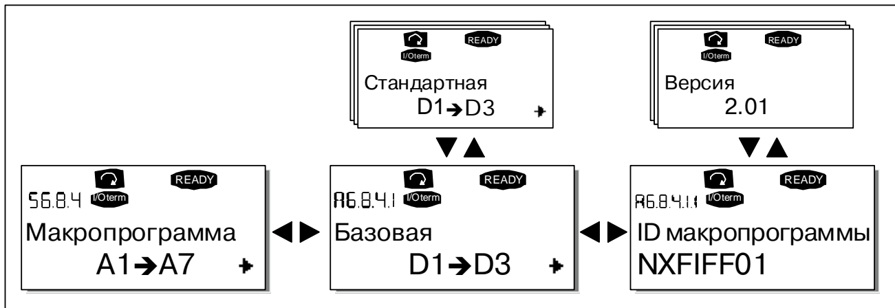
Рисунок 8-25. Информационное меню макропрограмм
