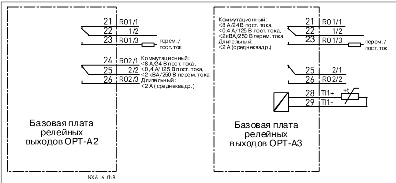
Рисунок 7-5. Принципиальная схема подсоединения базовых плат релейных выходов (OPT-A2/OPT-A3)
