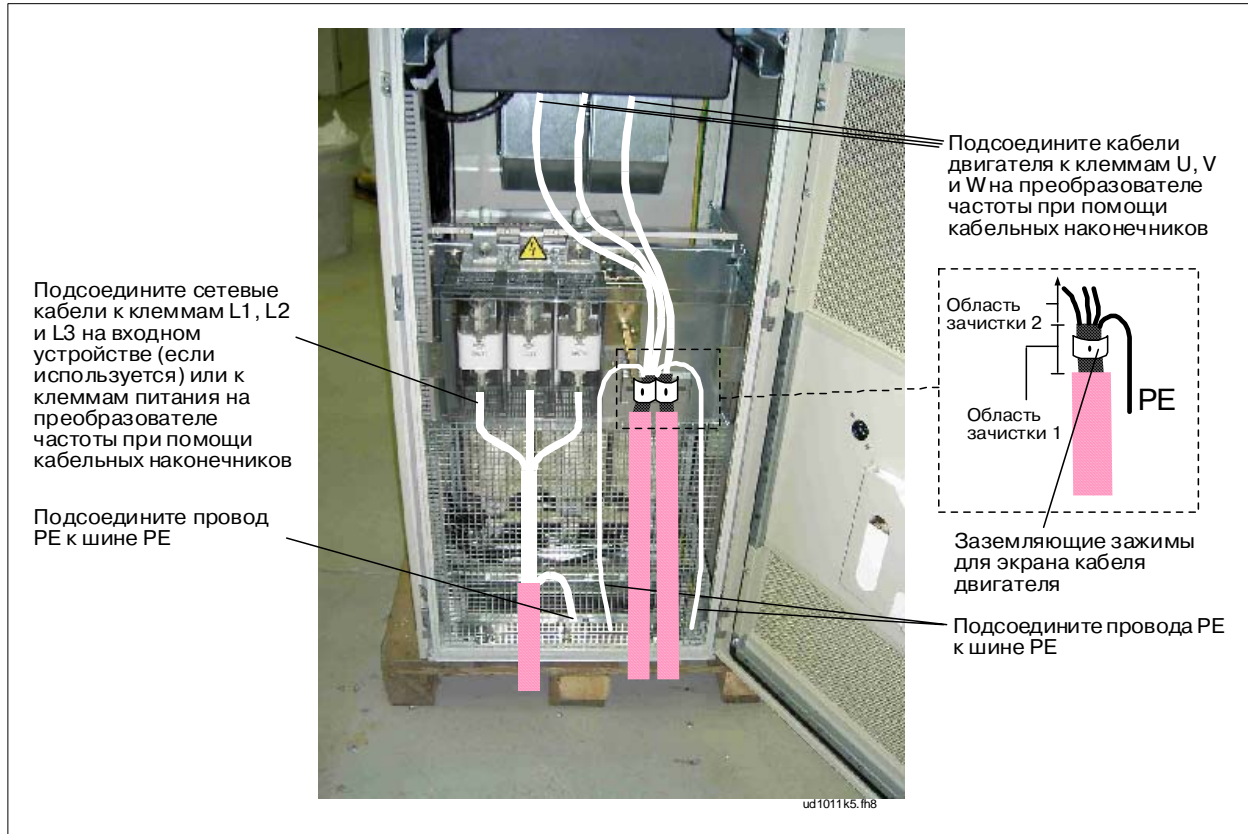
Рисунок 6-3. Прокладка кабелей питания, ввод кабеля снизу для типоразмеров FR10—FR12
