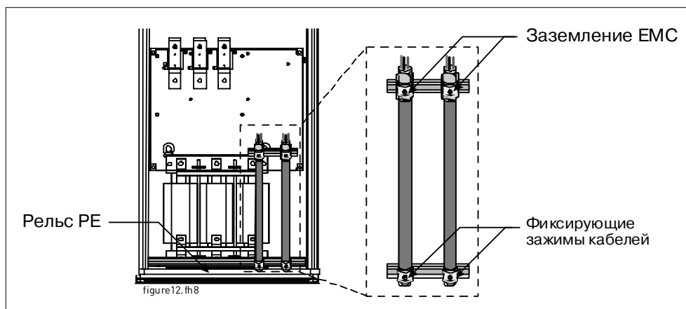
Рисунок 6-2. Установка электромагнитного заземления
