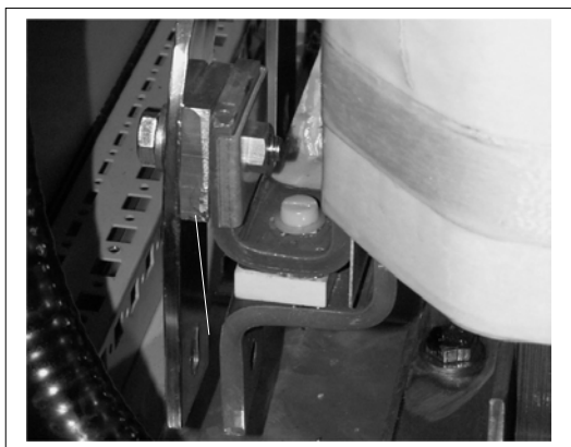
Рисунок 5-5. Входные дроссели
