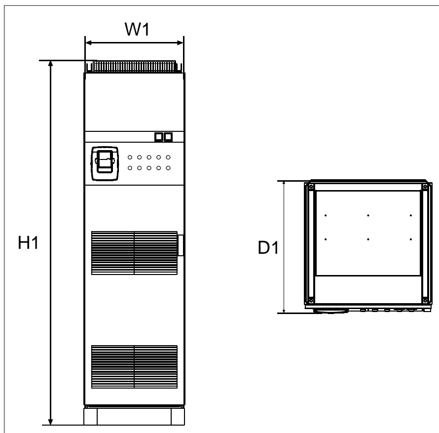
Рисунок 5-1. Габариты шкафа
