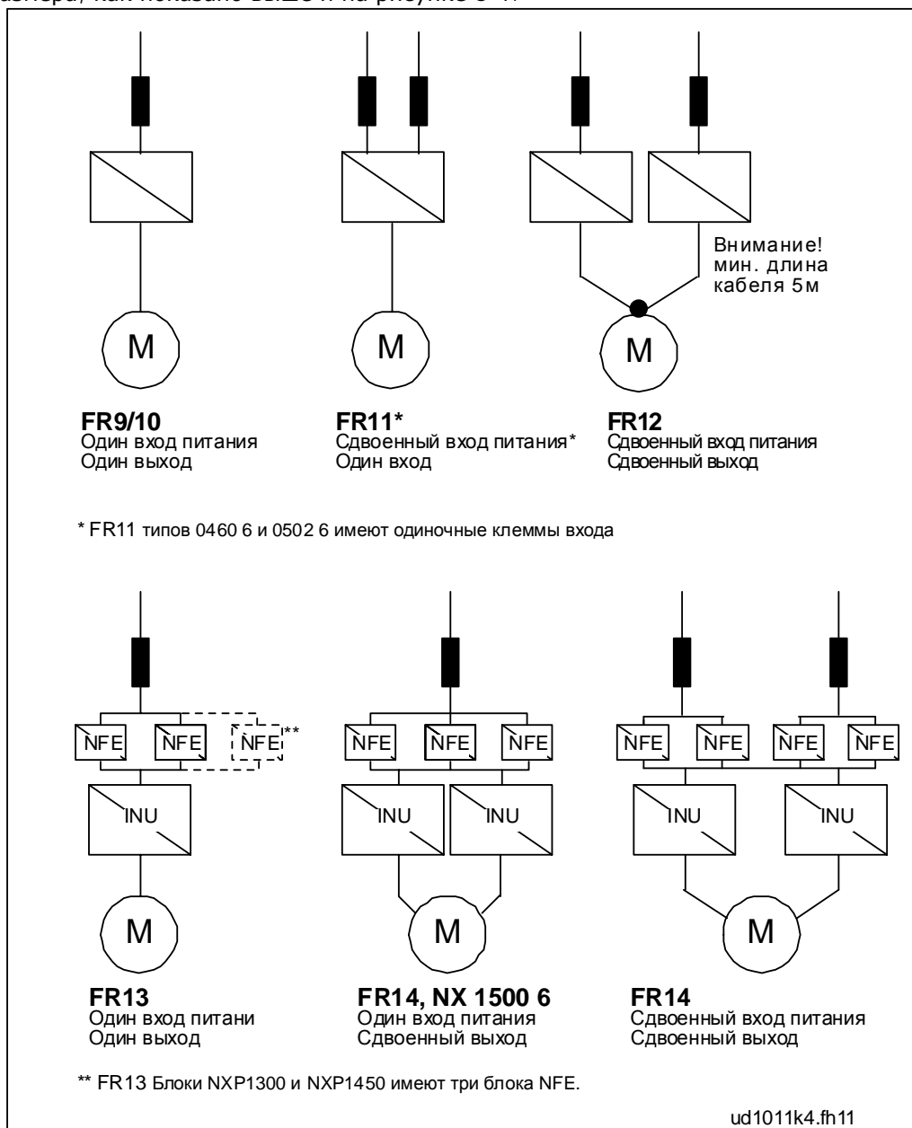
Рисунок 6-1. Схема типоразмеров FR10 – FR14, 6-пульсное питание
