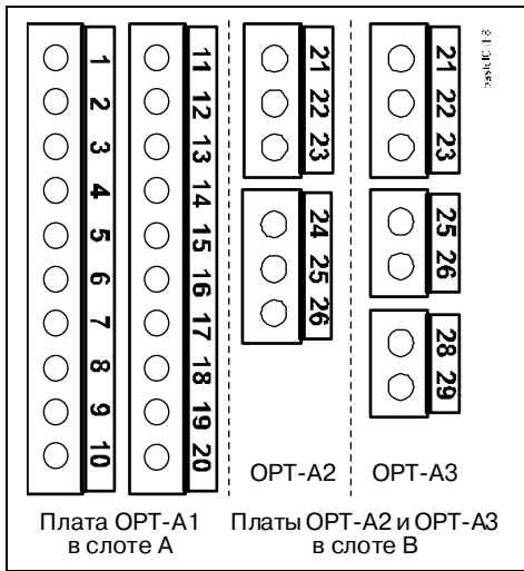
Рисунок 7-3. Клеммы входов/выходов базовых плат
