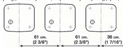
рис. 2 Монтаж нескольких сушилок
