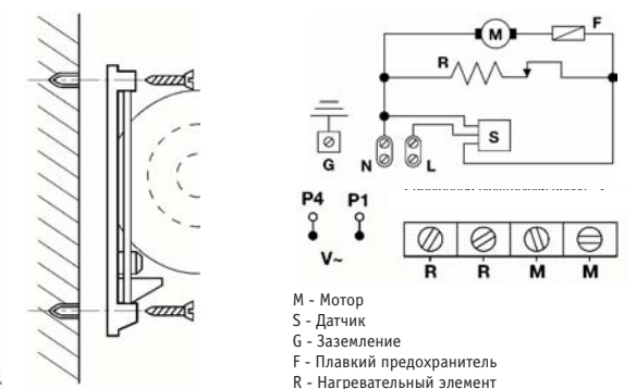
рис. 8 Монтаж сушилки на стену
