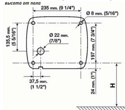
рис. 7 Монтажный шаблон
