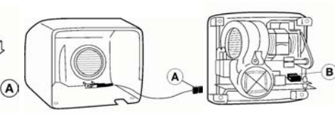
рис. 6 Подключение инфракрасного датчика
