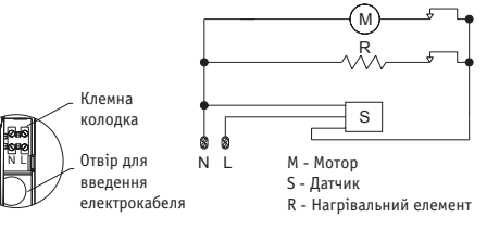
Мал. 7 Електросхема
