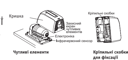
Мал. 3 Чутливі елементи
