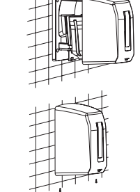
Мал. 8 Послідовність монтажу
