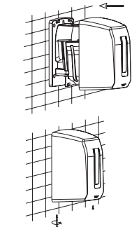
рис. 3 Последовательность монтажа
