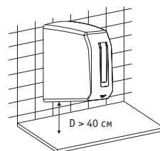
рис. 1 Минимальное расстояние до пола (или другой горизонтальной поверхности)
