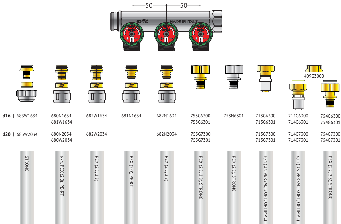
410N | Выходы 3/4" EK
