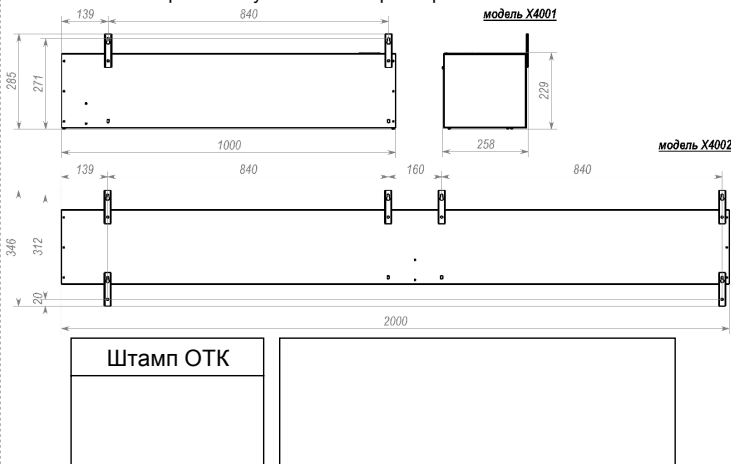
Рис. №1 Габаритные и установочные размеры завес X401A и X402A.
