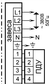
Схема подключения T206E, T209E, T212E, T218E, T309E, T318E к трёхфазной сети и ПДУ.
