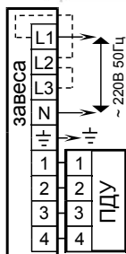
Схема подключения T206E к однофазной сети и ПДУ.
