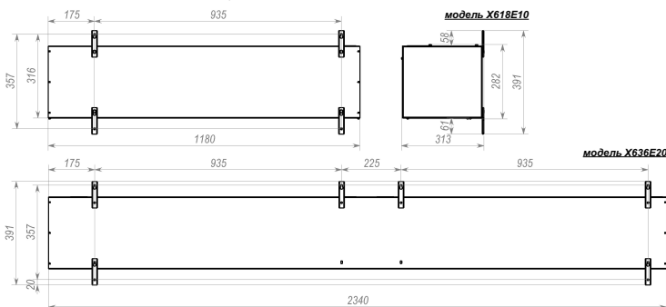
Рис. №1 Габаритные и установочные размеры завес X618E10 и X636E20.
