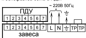
Схема подключения T103E Nova к однофазной сети и ПДУ.
