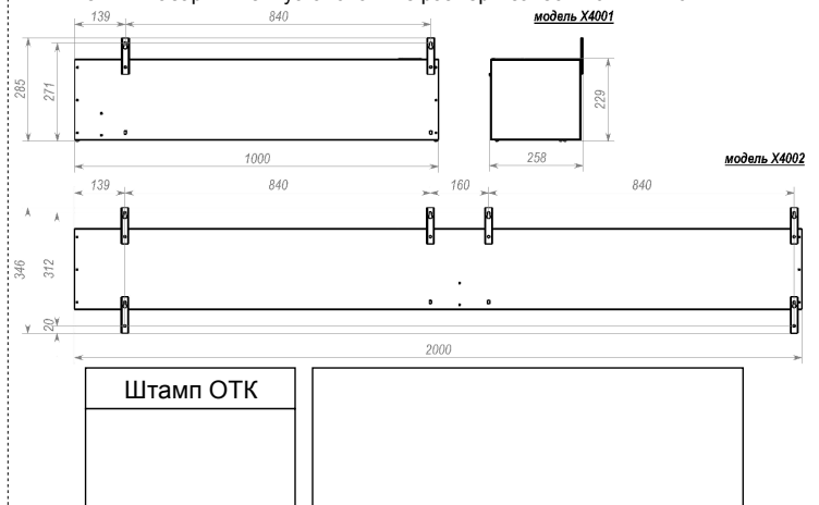
Рис. №1 Габаритные и установочные размеры завес X401A и X402A.
