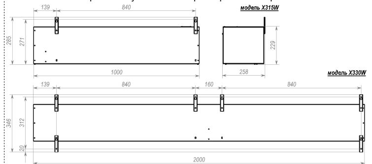
Рис. №1. Габаритные и установочные размеры завес серии Х300W.
