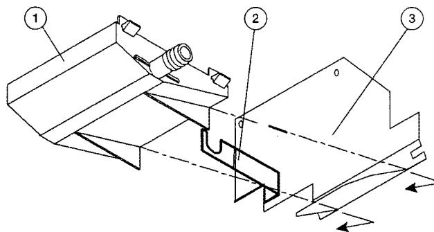
Рисунок 28 - Крепеж вспомогательного дренажного поддона
