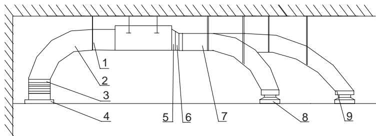
Монтаж круглого воздуховода
