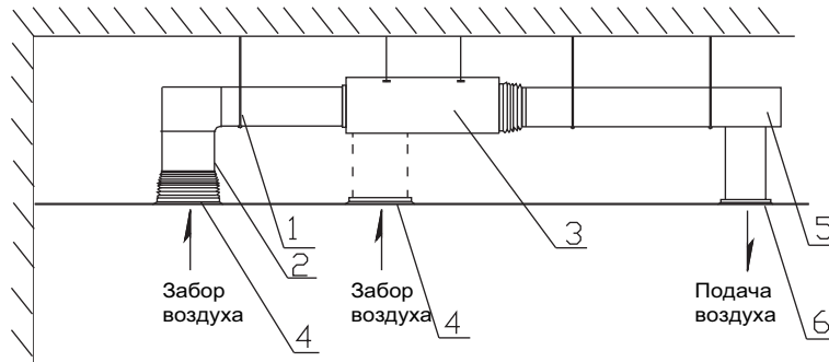
Монтаж прямоугольного воздуховода
