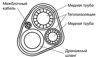
Монтажная пластина (на стене)
