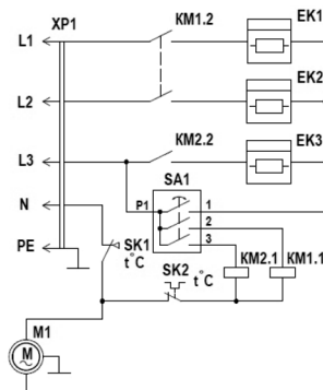
Схема коммутации переключателя SA1
