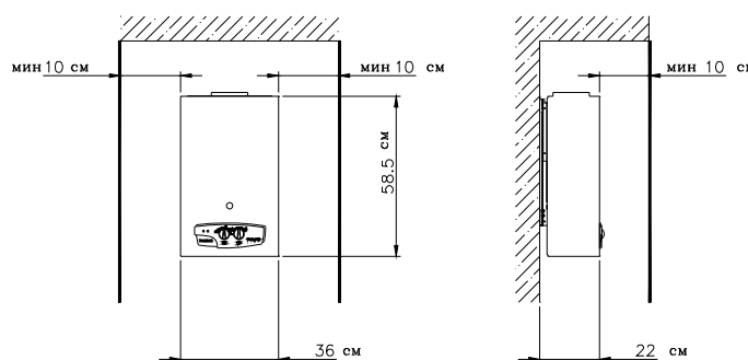
Рис. 3.3.1 Требуемые монтажные расстояния
