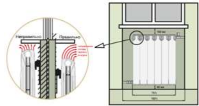
Схема установки радиатора
