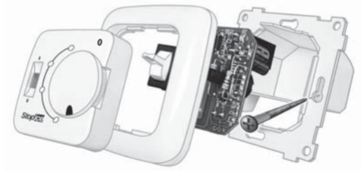
Рис. 3. Сборка терморегулятора
