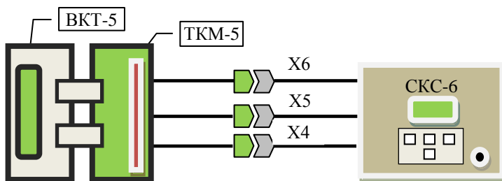
Рис. Б.2 Схема проверки BKT-5 с использованием SKC-6 и TKM-5 Разъемы X4...X6 (TKM-5) подключаются к одноименным разъемам стенда SKC6
