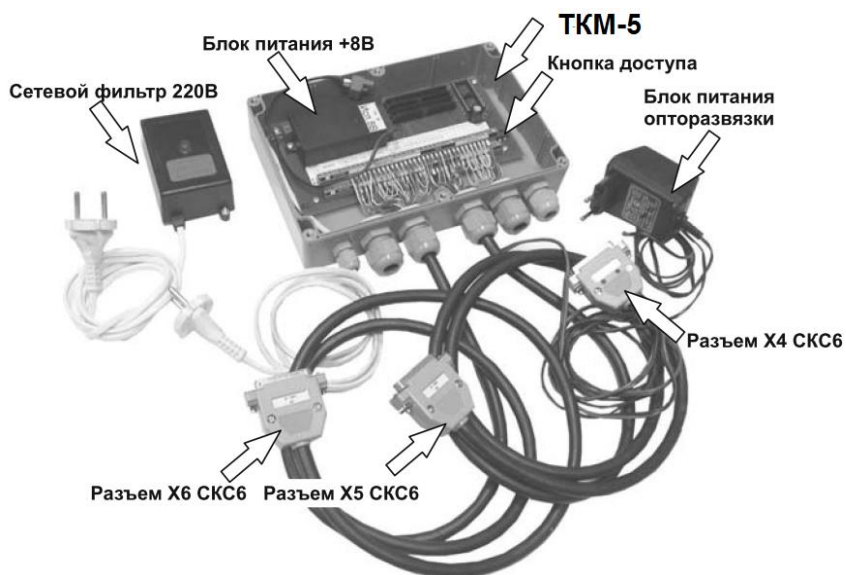
Рис. Б.3 Внешний вид TKM-5
