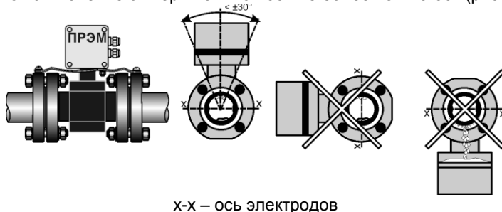
Рисунок 12 – Установка на горизонтальных каналах
