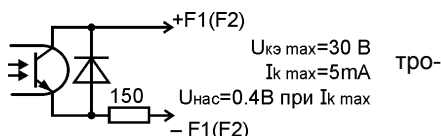
Рис. 6 – Схема выходного каскада
