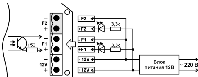
Рисунок 23 – Контроль выходных сигналов
