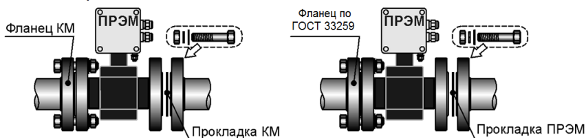
Рисунок 19 – Варианты монтажа ПРЭМ фланцевого исполнения
