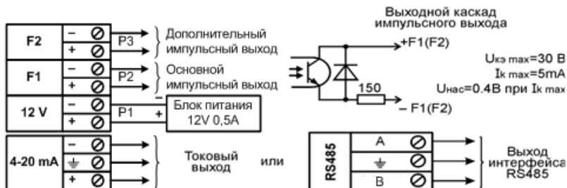
Рисунок 20 – Схема подключения ПРЭМ
