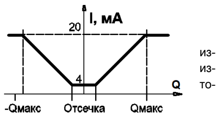
Рис. 5 – Выходная характеристика токового выхода ПРЭМ
