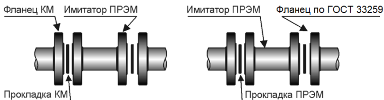
Рисунок 16 – Варианты установки габаритного имитатора ПРЭМ
