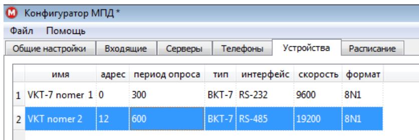
Рисунок 3.9 – Устройства
