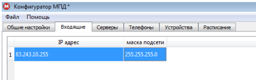
Рисунок 3.6 – Входящие
