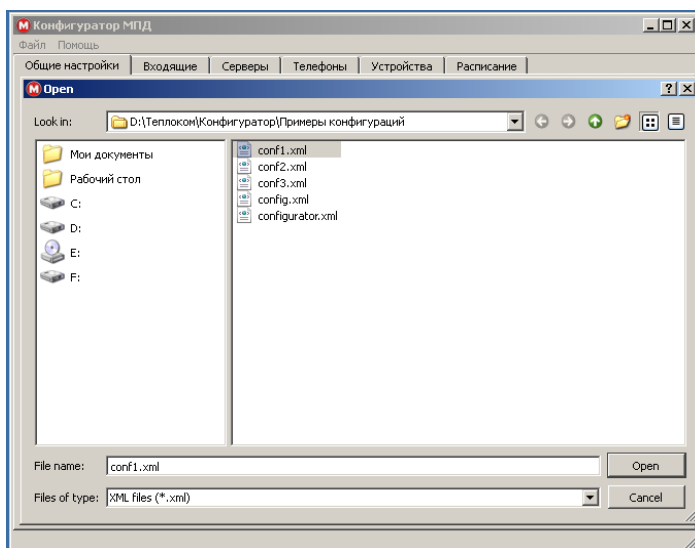
Рисунок 3.2 – Чтение конфигурации
