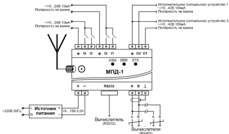
Рисунок 3.28 – Подключение
