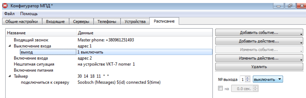
Рисунок 3.25 – Выход, выключение
