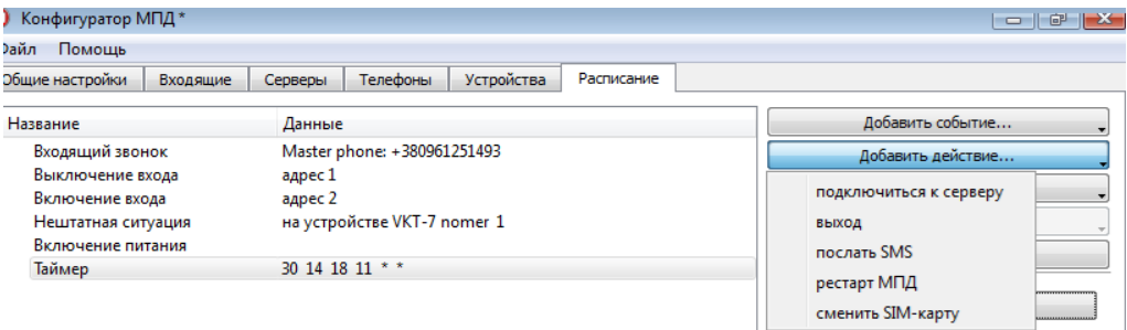
Рисунок 3.21 – Действия
