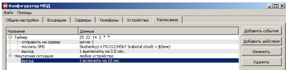
Рисунок 4.1 – Пример конфигурации
