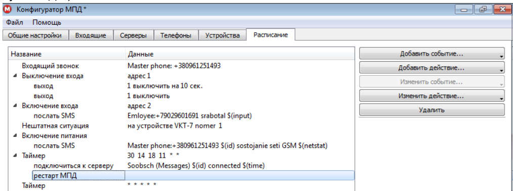
Рисунок 3.27 – Рестарт
