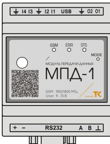
Рисунок 2.1 – Внешний вид
