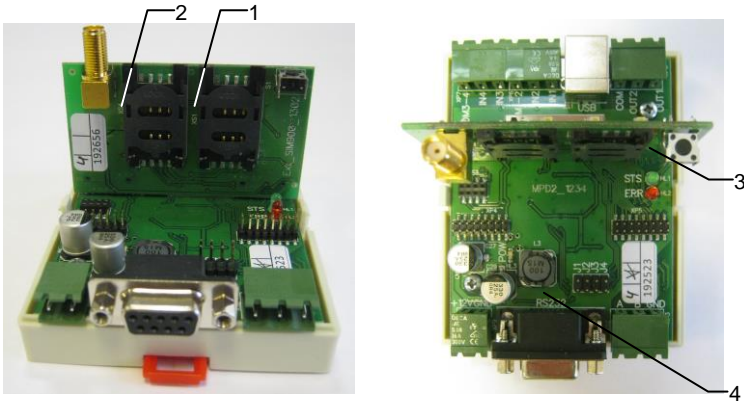
Рисунок 2.4 – Устройство
