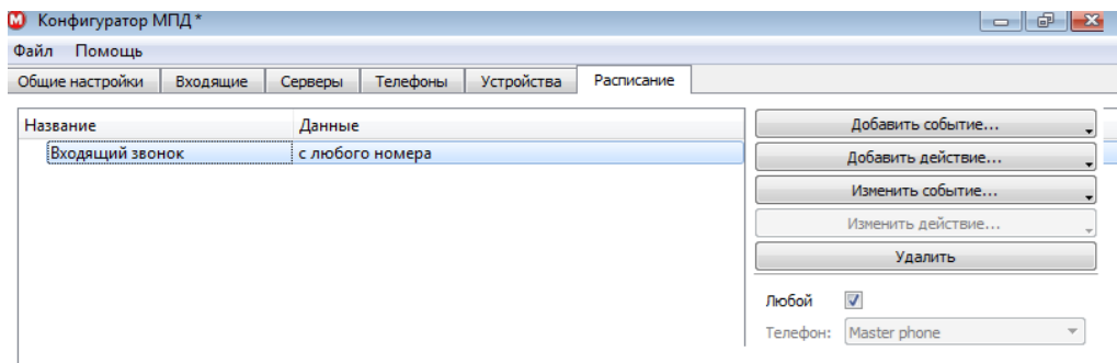
Рисунок 3.17 – Входящий звонок
