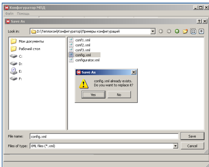
Рисунок 3.3 – Запись конфигурации
