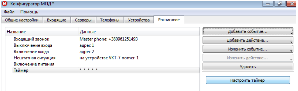
Рисунок 3.11 – Настройка таймера
