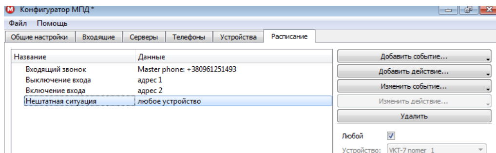
Рисунок 3.19 – Нештатная ситуация
