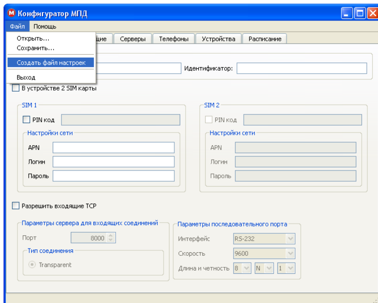
Рисунок 3.1 – Создание файла
