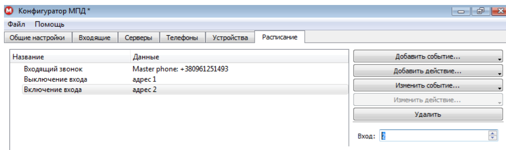
Рисунок 3.18 – Вход
