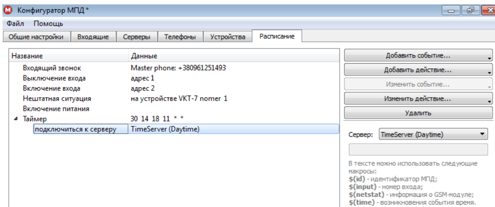
Рисунок 3.22 – Сервер
