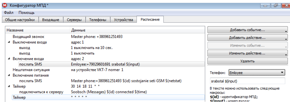
Рисунок 3.23 – SMS
