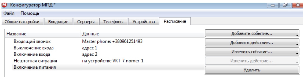
Рисунок 3.16 – Включение питания
