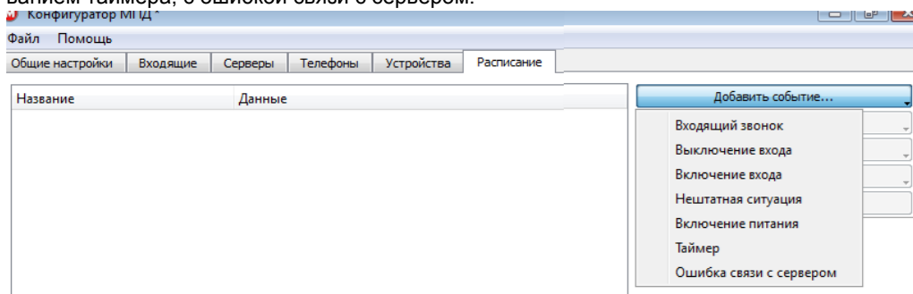
Рисунок 3.10 – События
