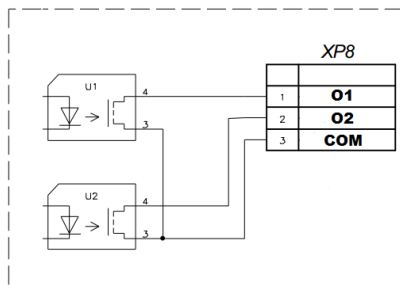
Рисунок 2.3 – Цифровые выходы
