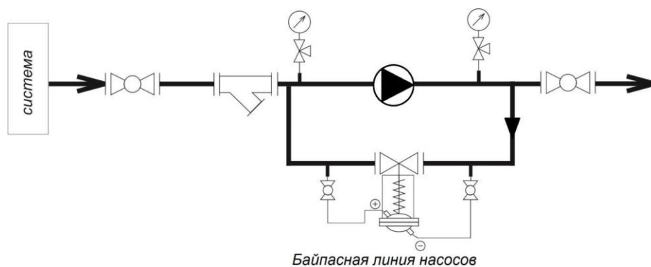
Рисунок А.2-Схема подключения регулятора
