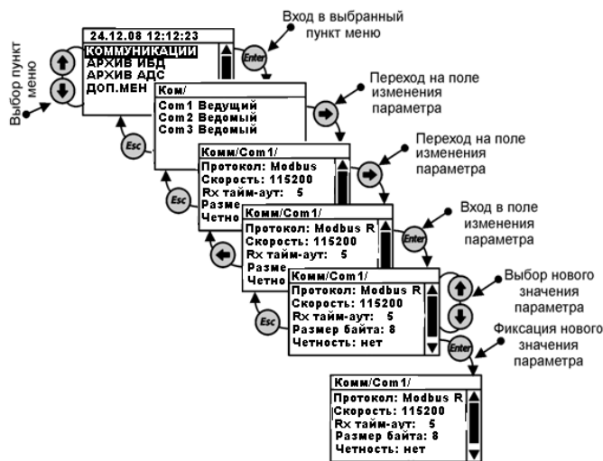
Рис. 1.5.6.7.18.1 Общее меню раздела «Коммуникации»
