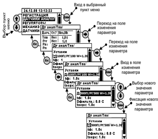
Рис. 1.5.6.7.1 Общее меню раздела «Датчики аналоговые»
