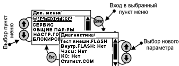
Рис. 1.5.6.21.1 Общее меню раздела «Доп меню» диагностика
