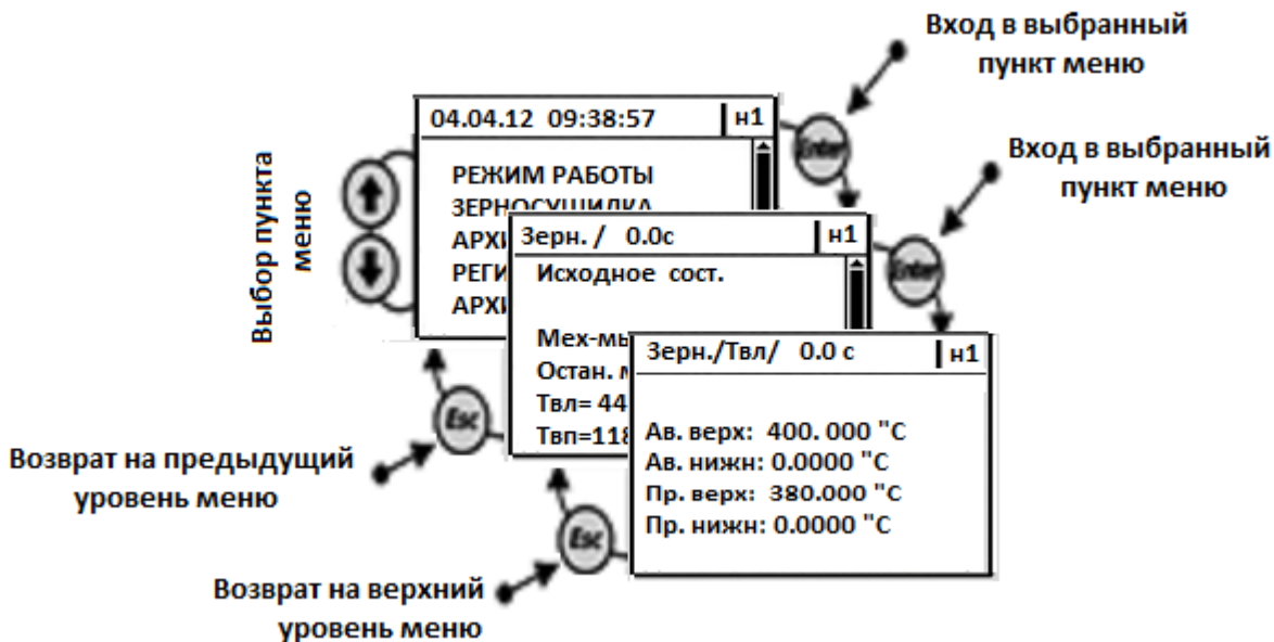
Рис. 1.5.6.2.1 Общее меню раздела «Зерносушилка»
