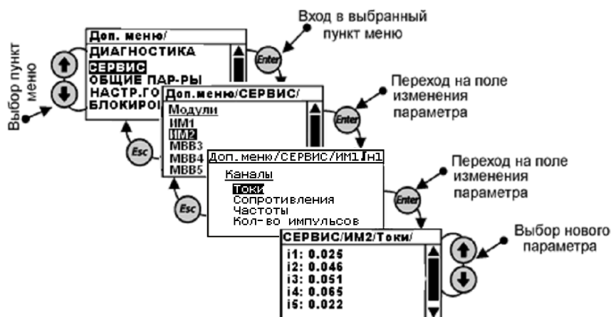
Рис. 1.5.6.21.2 Общее меню раздела «Доп меню» сервис
