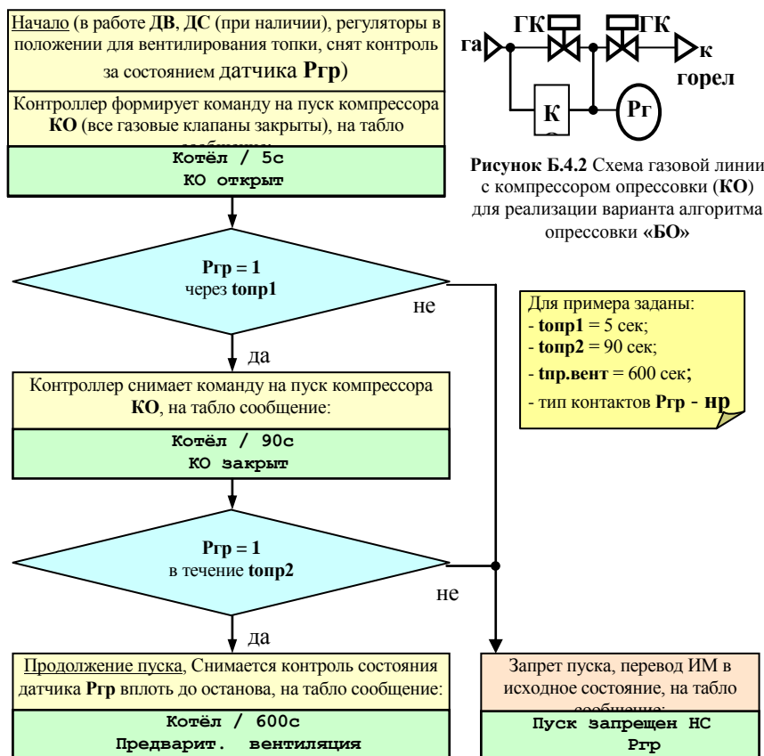
Рисунок Д.4.1 Блок-схема алгоритма варианта опрессовки «БО» с компрессором КО
