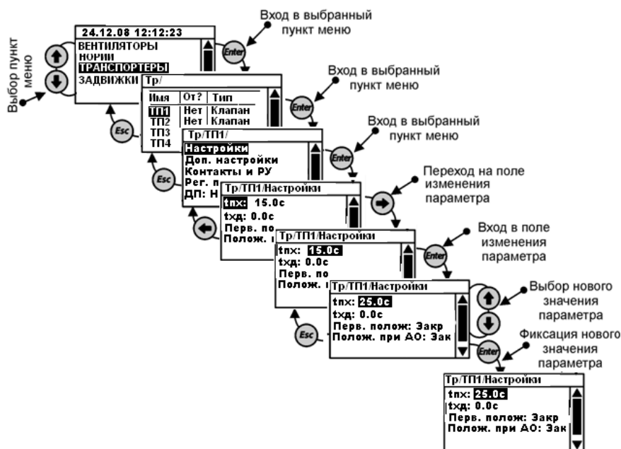
Рис. 1.5.6.11.1 Общее меню раздела «Транспортеры»
