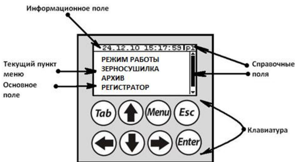
Рис.1.4.3.1 Табло контроллера
