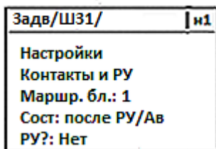
Рис. 1.5.6.12.2 Меню раздела «Задвижки» характеристики механизма
