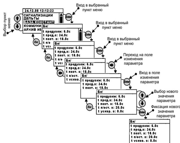
Рис1.5.6.16.1 Общее меню раздела «База констант»
