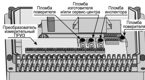
Рисунок 2 – Места пломбирования ПРИЗ в корпусном исполнении
