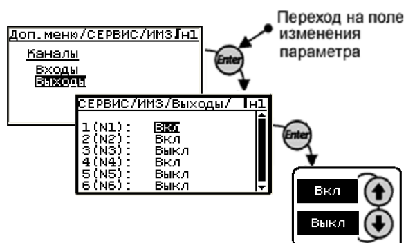
Рис. 1.5.6.21.2.8 Общее меню раздела «Доп меню»-> сервис-> MBV-> Выходы
