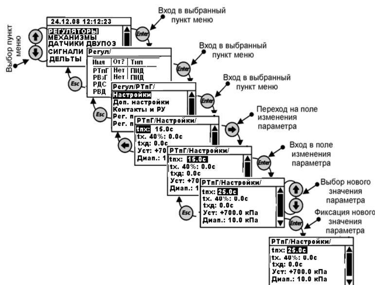
Рис. 1.5.6.8.1 Общее меню раздела «Регуляторы»
