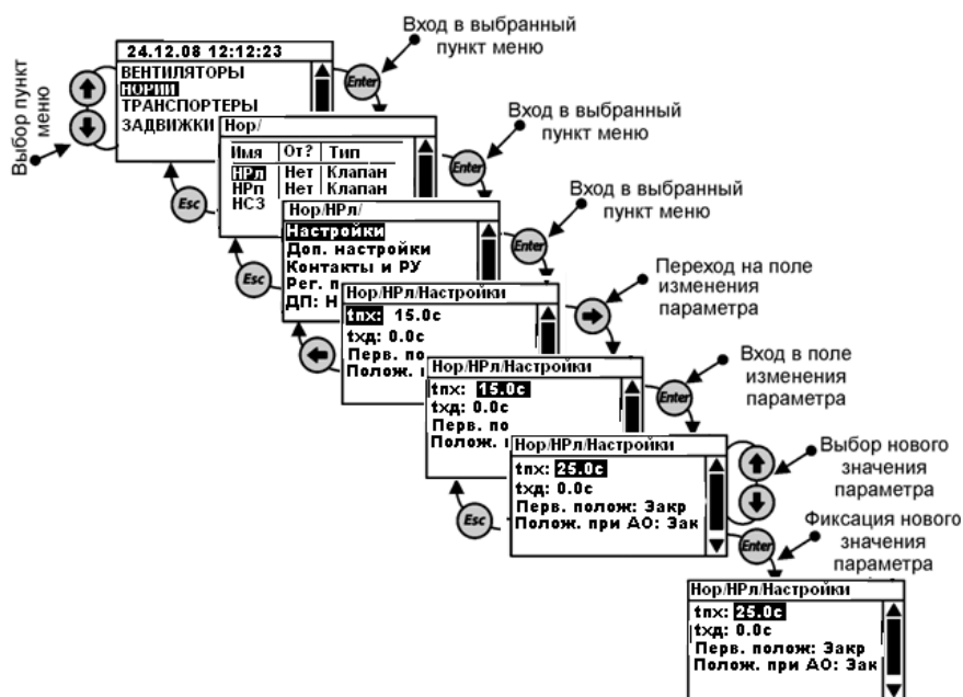
Рис. 1.5.6.10.1 Общее меню раздела «Нории»
