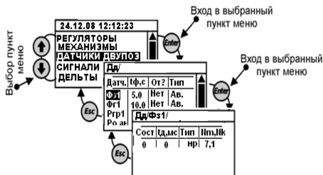
Рис. 1.5.6.15.1 Общее меню раздела «Датчики двухпозиционные»
