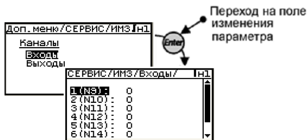
Рис. 1.5.6.21.2.7 Общее меню раздела «Доп меню»-> сервис-> MBV-> Входы
