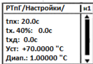
Рис. 1.5.6.8.3 Меню раздела «Регуляторы» настройки регулятора
