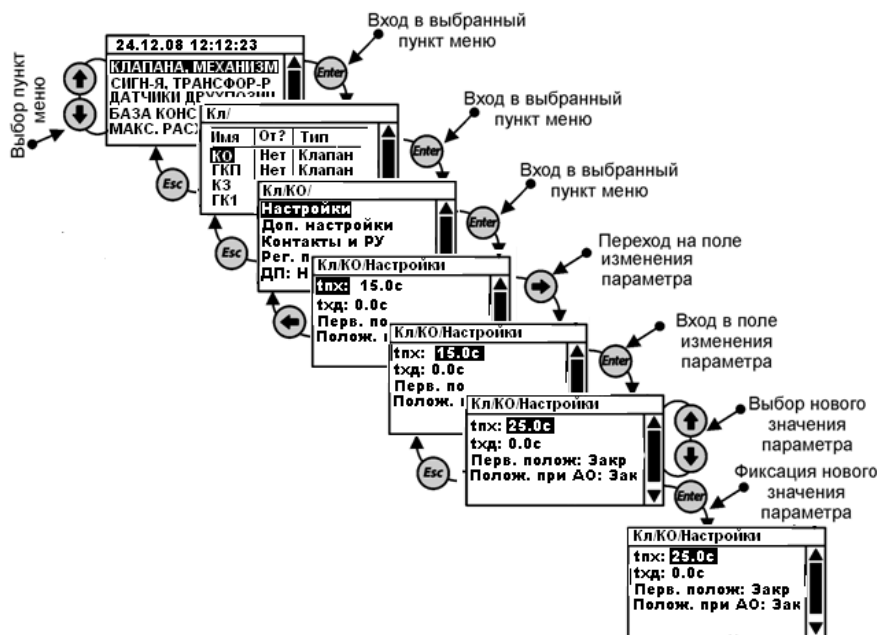
Рис. 1.5.6.13.1 Общее меню раздела «Клапана, механизмы»
