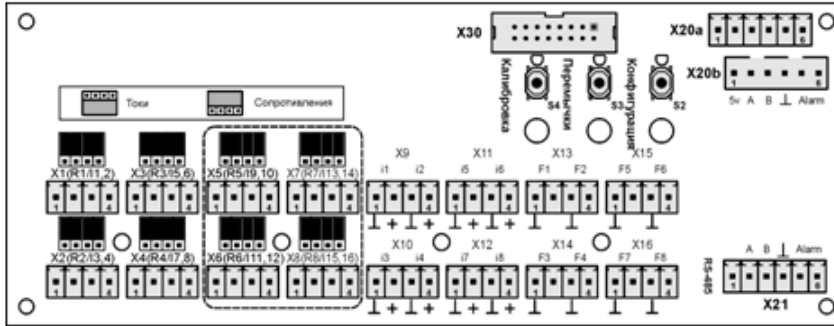
Рис. В.1 – Схема расположения разъемов ПРИЗ-1-Х
