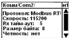
Рис. 1.5.6.18.3 Меню раздела «Коммуникации» характеристики Com-портов
