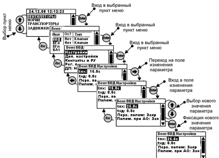
Рис. 1.5.6.9.1 Общее меню раздела «Вентиляторы»
