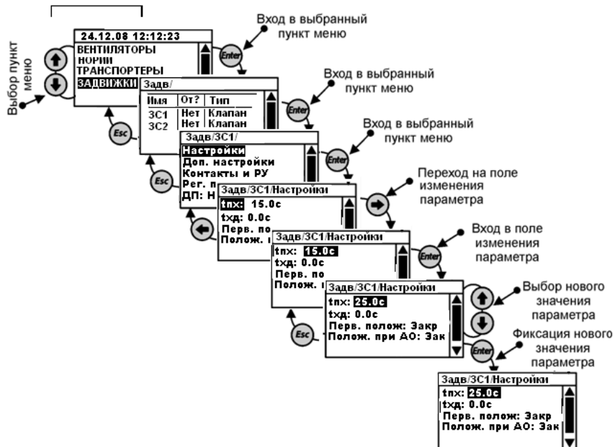
Рис. 1.5.6.12.1 Общее меню раздела «Задвижки»
