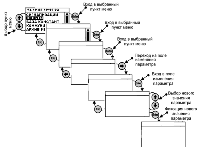
Рис. 1.5.6.17.1 Общее меню раздела «Дельты»
