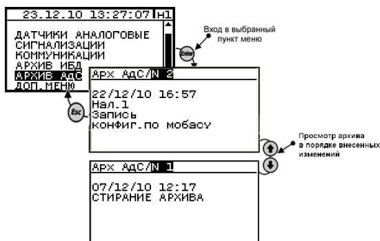
Рис. 1.5.6.20.1 Общее меню раздела «Архив АдС»
