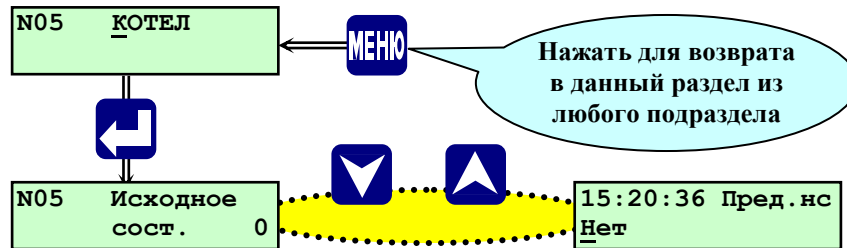
Рисунок 6.6.1.1 Раздел основного меню «Котел»
