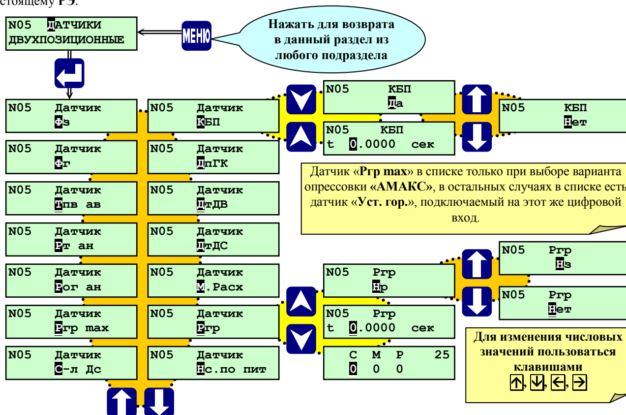
Рисунок 6.6.11.1 Раздел основного меню наладчика «Датчики двухпозиционные» (водогрейный котел)
