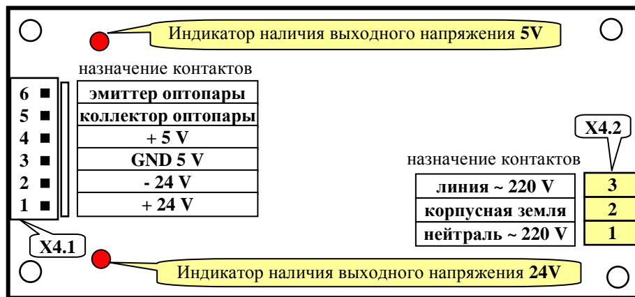
Рисунок А.5.4 - Плата БП (блока питания) контроллера
