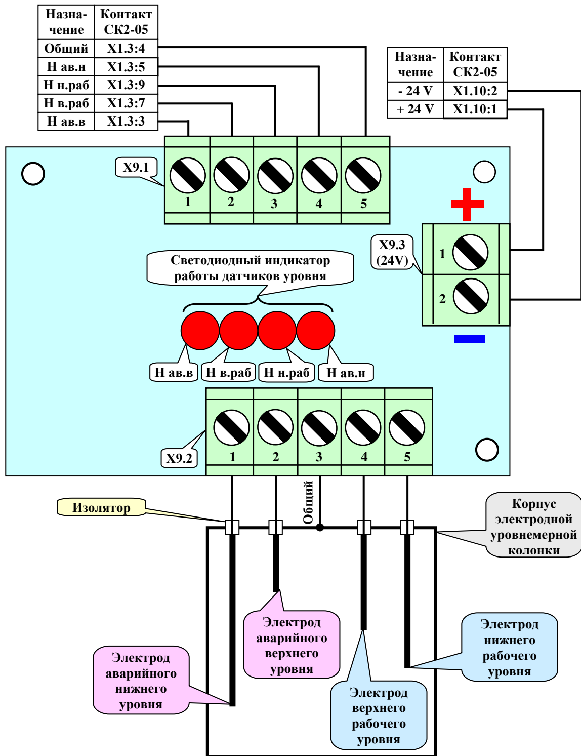
Рисунок А.5.7 - Подключение платы УК (уровнемерной колонки) и нумерация её разъёмов
