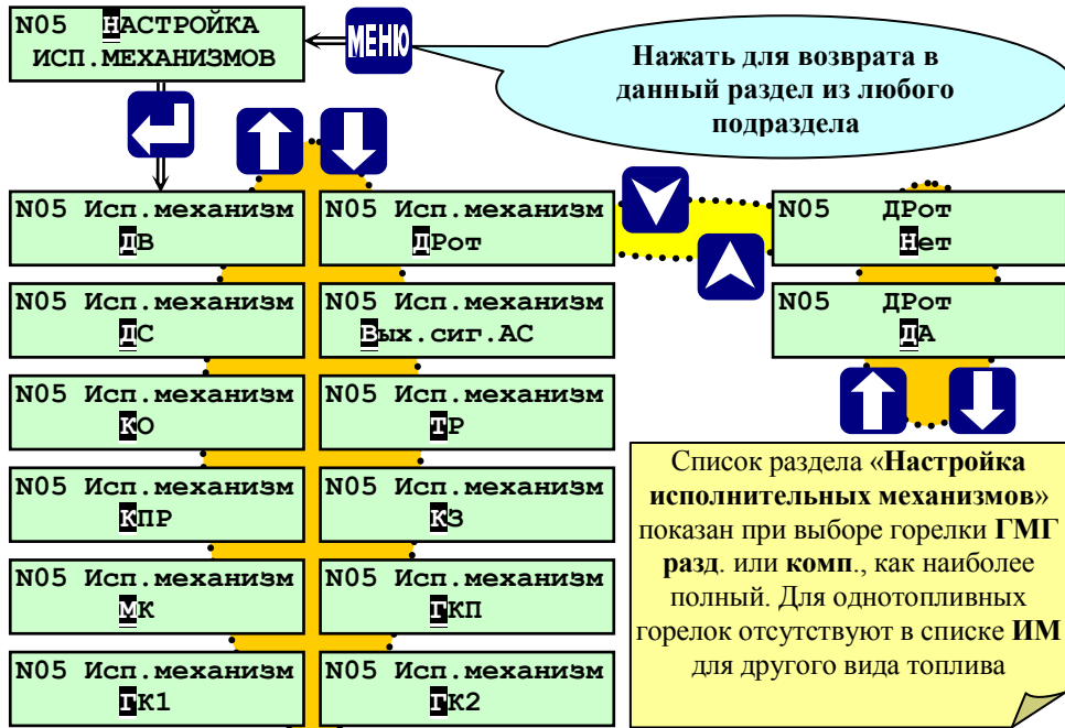
Рисунок 6.6.12.1 Раздел основного меню наладчика «Настройка исполнительных механизмов»
