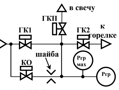
Рисунок Б.3.2 Схема газовой линии для реализации алгоритма опрессовки «АМАКС»
