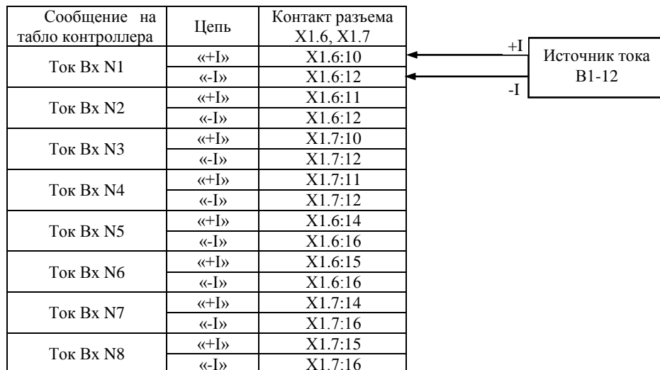
Рисунок Д.2.2 - Схема подключения источника тока при настройке IBI , при поверке токовых входов
