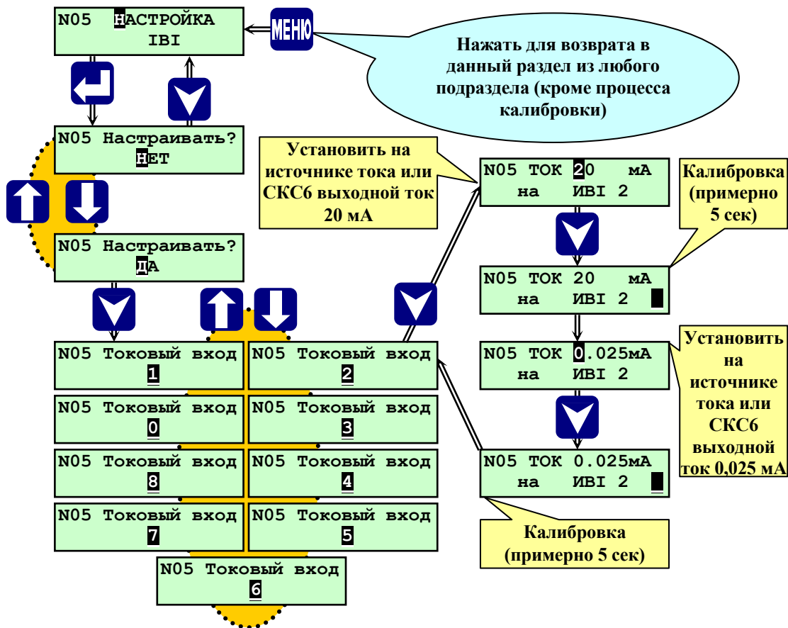
Рисунок 6.6.14.1 Раздел основного меню наладчика « Настройка ИВИ »
