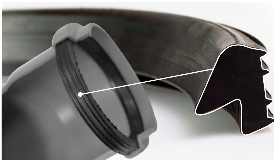
ТРУБА КАНАЛИЗАЦИОННАЯ С РАСТРУБОМ
