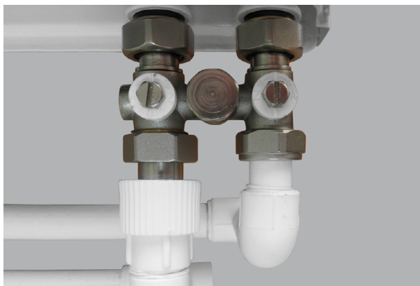
Сравнительное соединение с применением комбинированной муфты и штуцера-евроконуса
