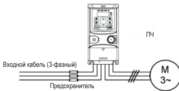
Рис. 3-14: Расположение предохранителей
