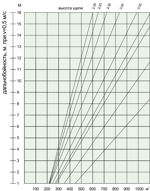
Дальность приточной струи
