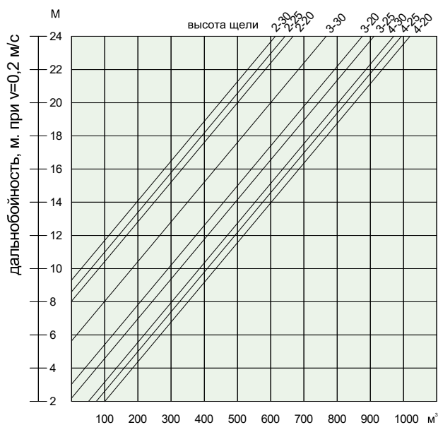
Дальность приточной струи
