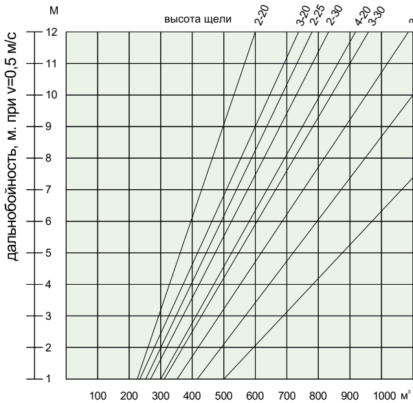
Дальнобойность приточной струи
