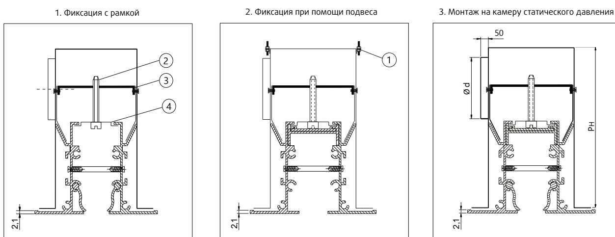
Рис. 4. Варианты монтажа
