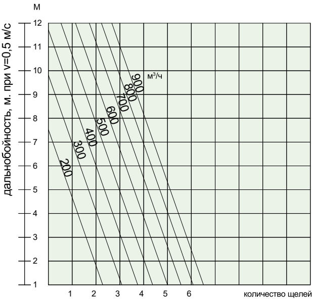
Дальнобойность приточной струи щелевого диффузора A-Line-H-20-T2 с КСД при длине A=1000 мм подача воздуха, угол наклона ламели \alpha = 0^\circ
