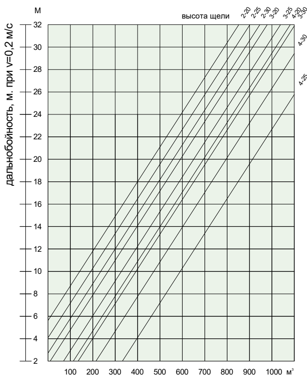
Дальность приточной струи
