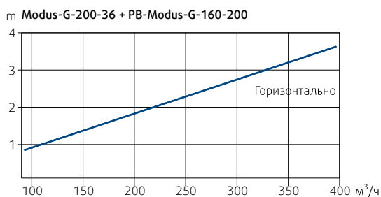
Диаграмма 6: Дальность броска изотермической струи (горизонтальная подача воздуха) при конечной скорости 0,2 м/с
