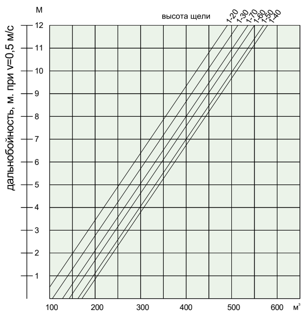
Дальнобойность приточной струи
