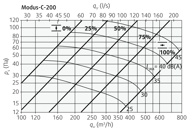
Перепад давления &amp; A-взвешенный уровень звуковой мощности
