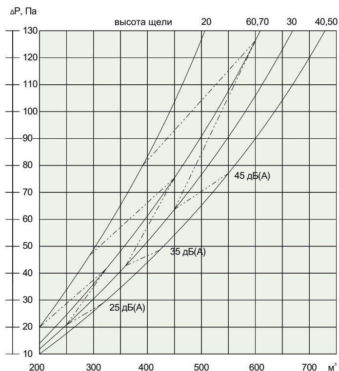
Уровень звуковой мощности и падение давления
