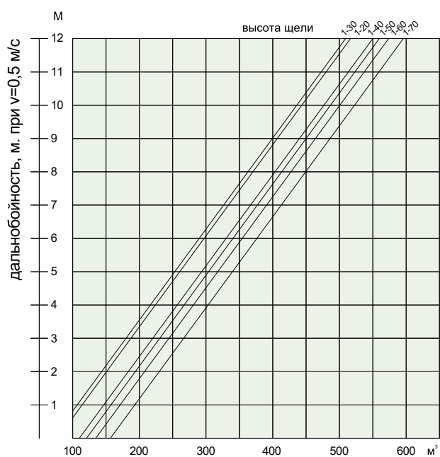
Дальность приточной струи
