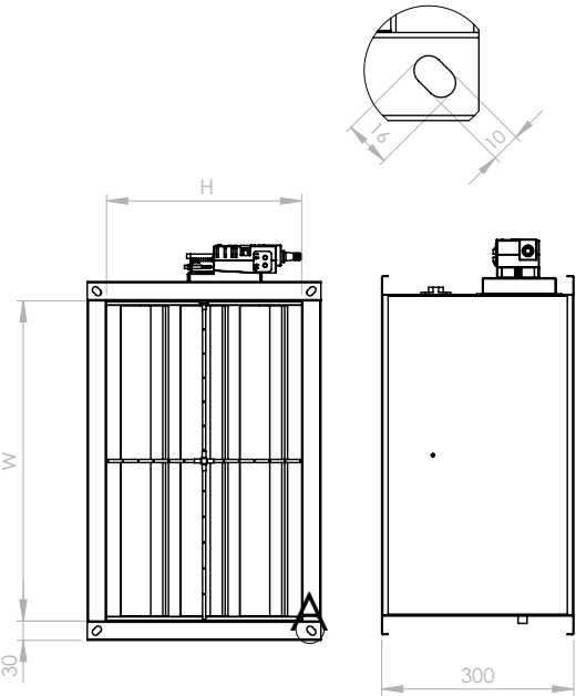
Рис. 3. Исполнение без шумоизоляции
