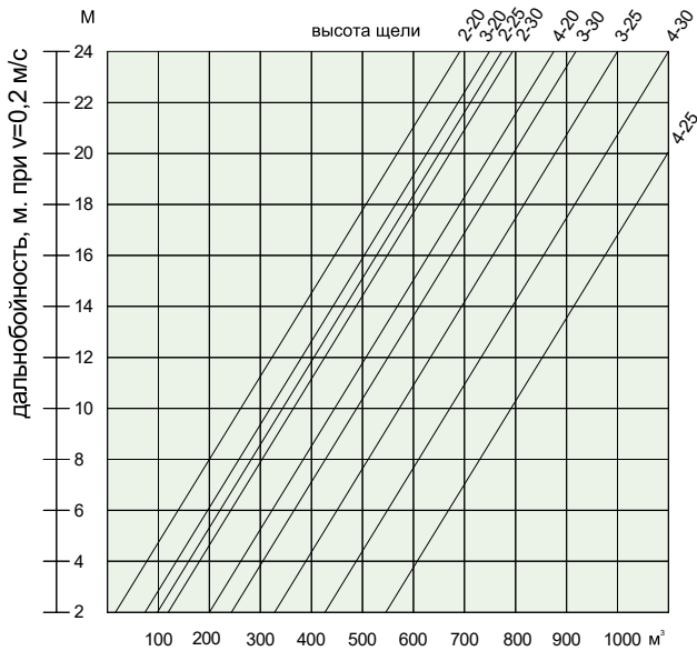
Дальнобойность приточной струи
