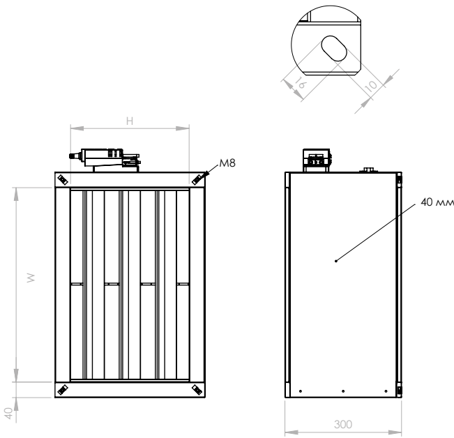
Рис. 4. Шумоизолированное исполнение
