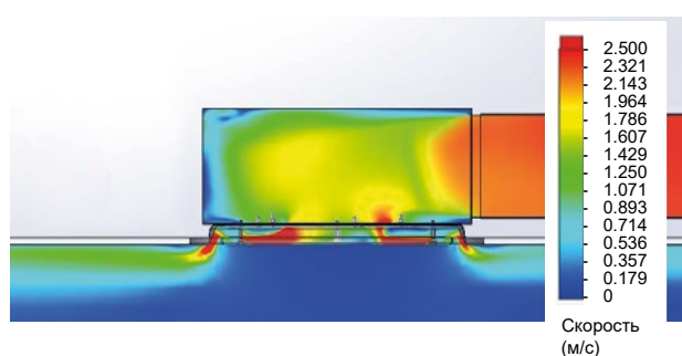
Скорость потока в сечении диффузора
