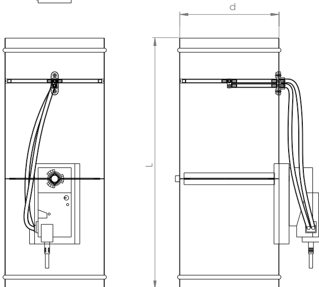
Рис. 1. Исполнение без шумоизоляции
