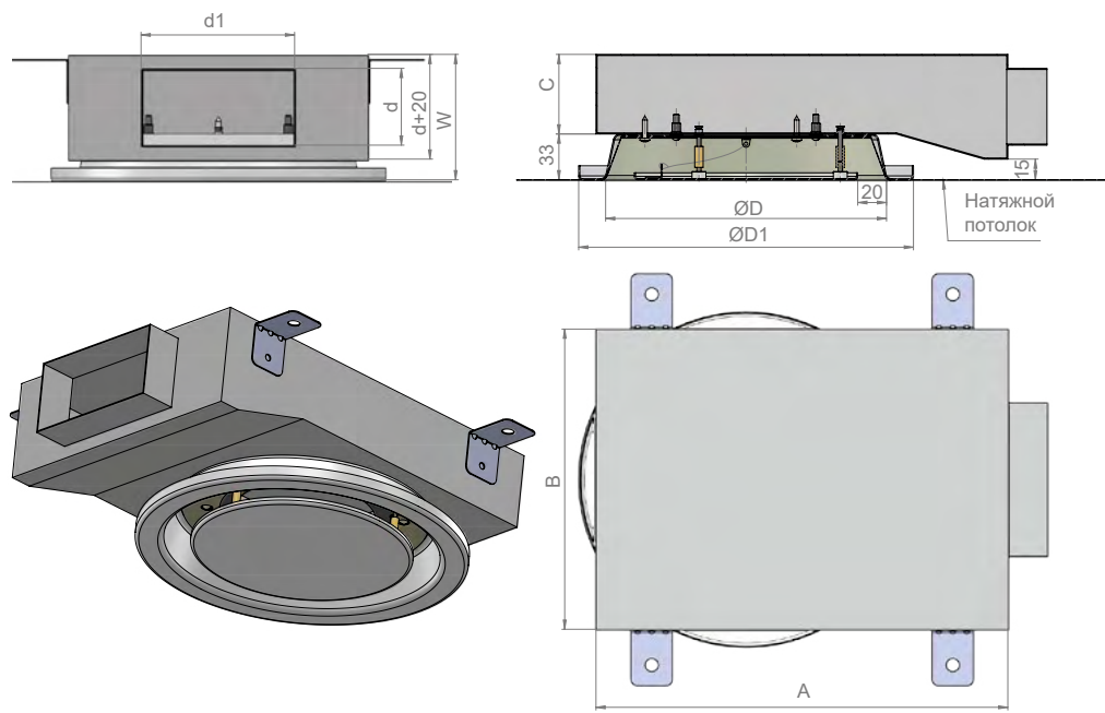
Габаритно-посадочные размеры диффузора NTP с уменьшенной камерой статического давления с прямоугольной врезкой РВ-U-Р
