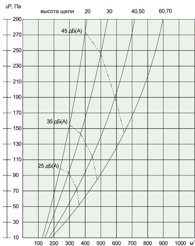
Уровень звуковой мощности и падение давления
