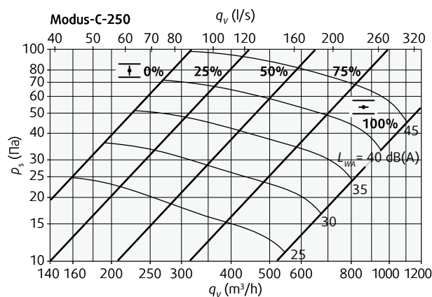
Перепад давления &amp; A-взвешенный уровень звуковой мощности
