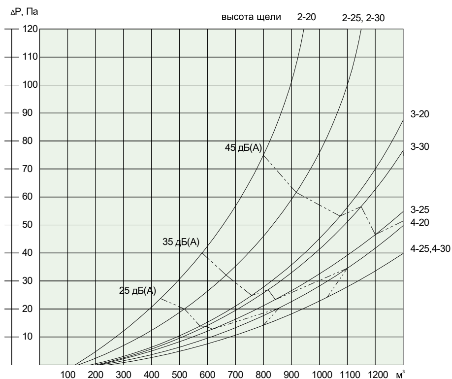
Уровень звуковой мощности и падение давления
