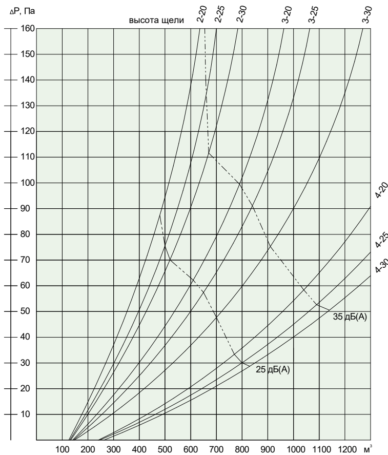
Уровень звуковой мощности и падение давления
