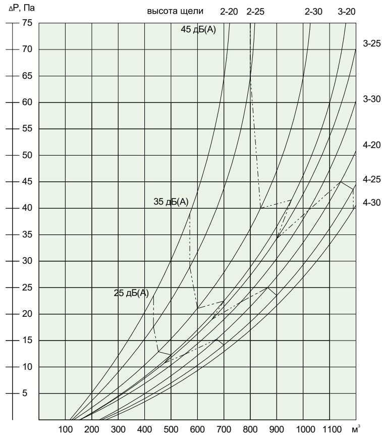
Уровень звуковой мощности и падение давления
