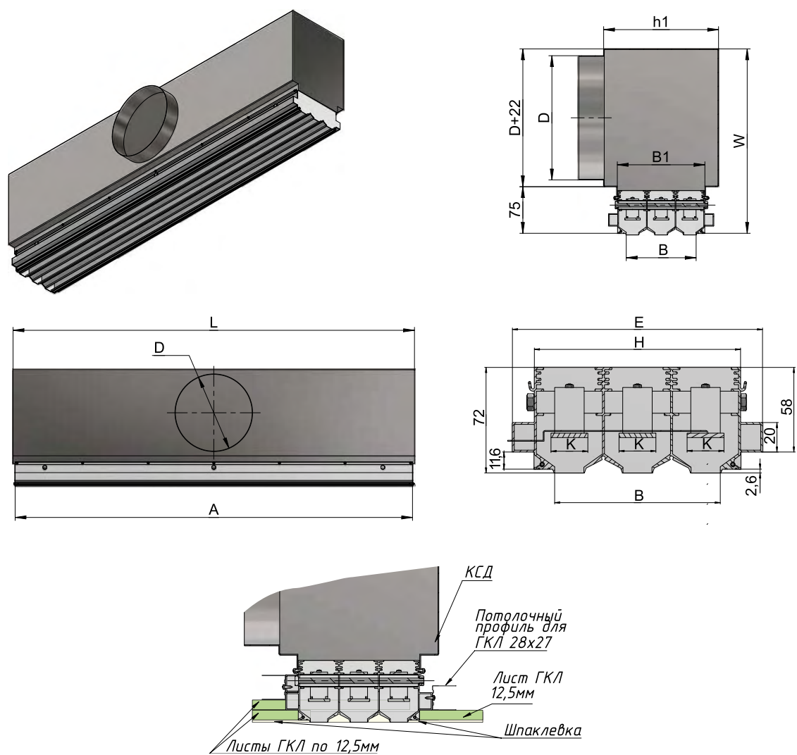
Габаритно-посадочные размеры щелевого диффузора + КСД стандартной конфигурации АхВ размеры видимой части диффузора после монтажа А – ширина щелей, В – высота щелей
