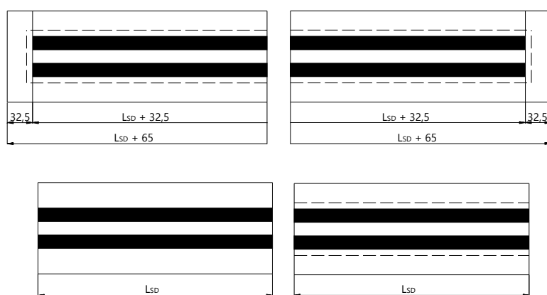
Рис. 3. Длины диффузоров
