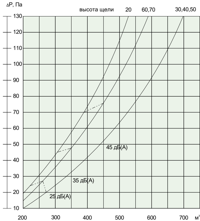
Уровень звуковой мощности и падение давления
