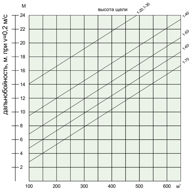
Дальнобойность приточной струи
