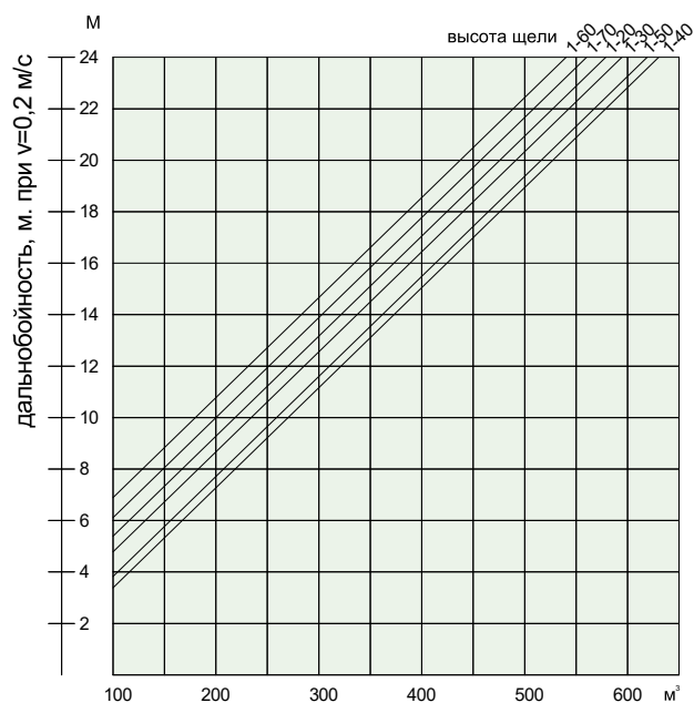
Дальнобойность приточной струи
