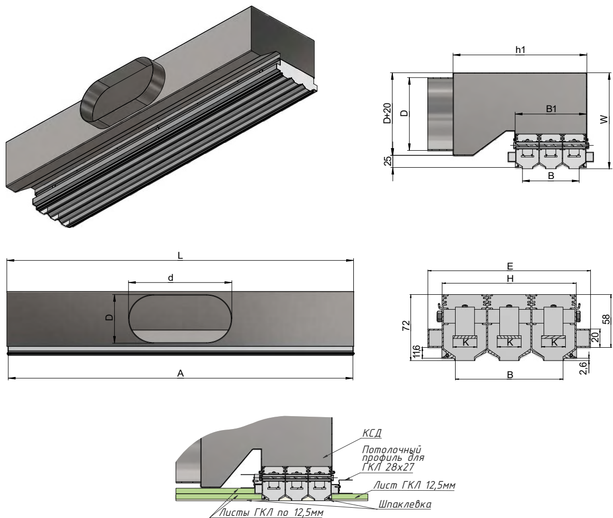
Габаритно-посадочные размеры щелевого диффузора + уменьшенная КСД-U-0 с овальной вырезкой А — ширина щелей, В — высота щелей
