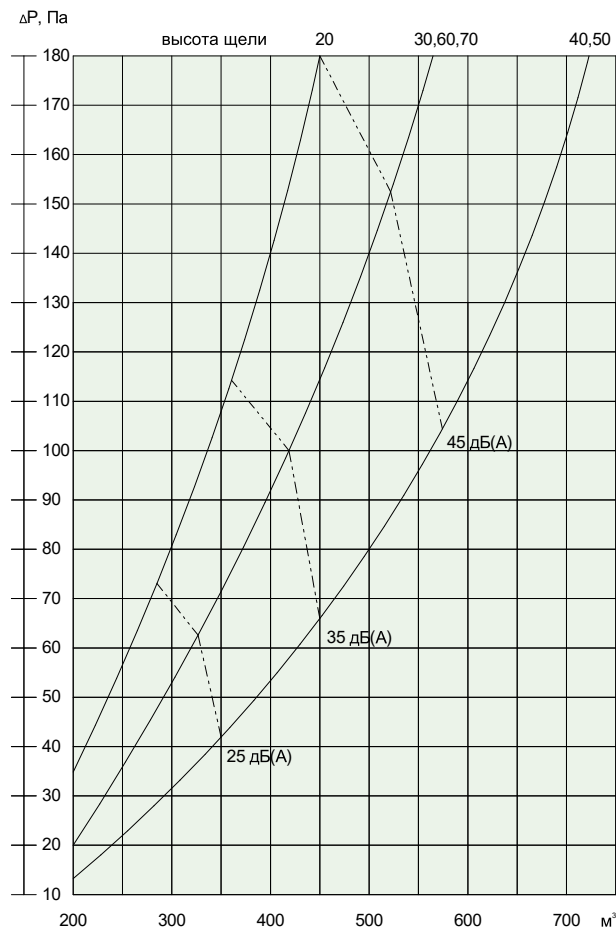
Уровень звуковой мощности и падение давления
