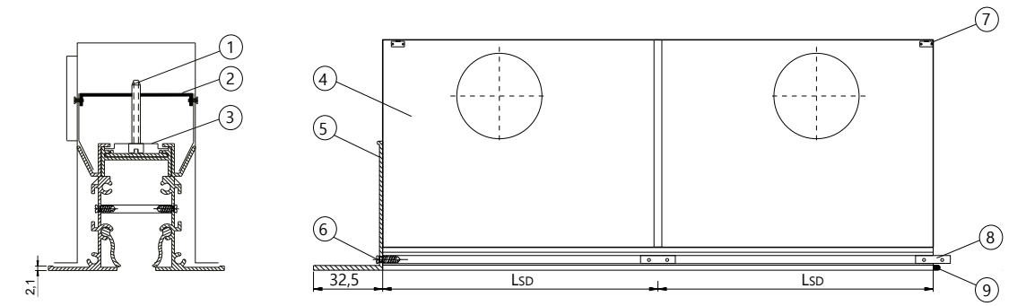
Рис. 5. Монтаж диффузоров в линию
