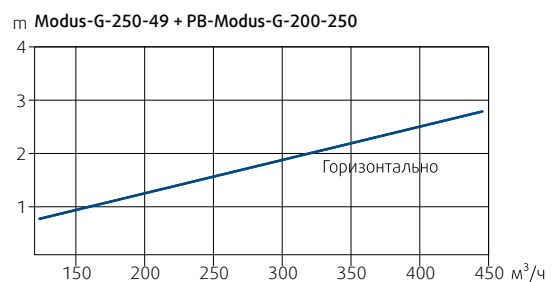
Диаграмма 7: Дальность броска изотермической струи (горизонтальная подача воздуха) при конечной скорости 0,2 м/с
