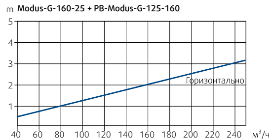
Диаграмма 4: Дальность броска изотермической струи (горизонтальная подача воздуха) при конечной скорости 0,2 м/с
