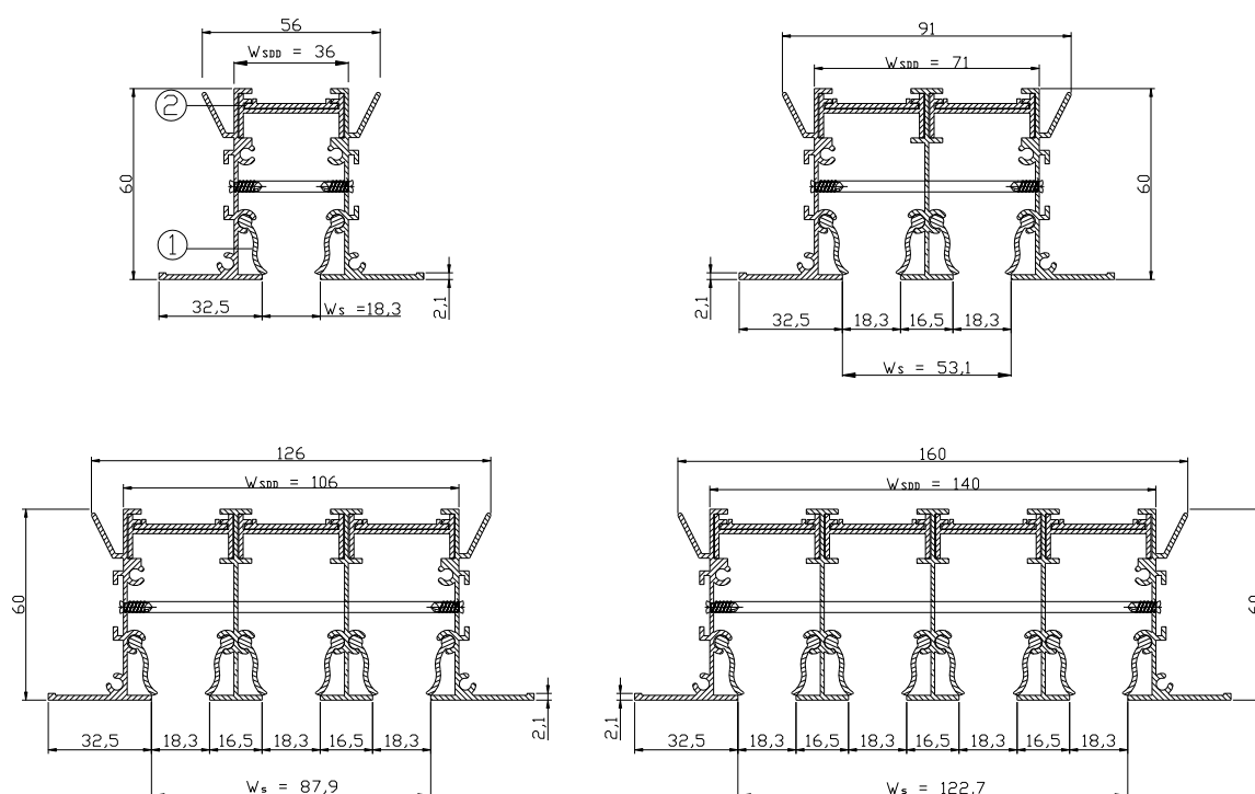
Рис. 1. Размеры приточного щелевого диффузора (1-2-3-4 слота)
