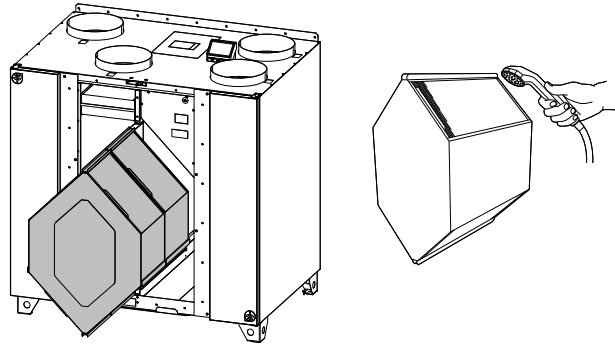
Рис. 7 Снятие и чистка теплообменника
