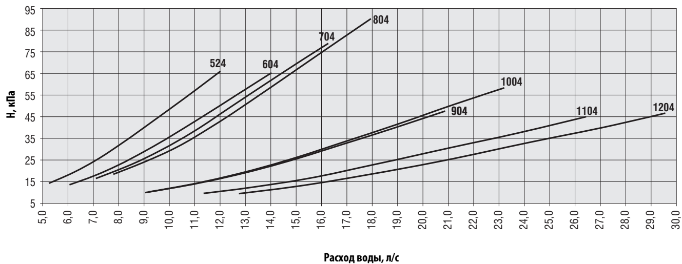
АГРЕГАТЫ WQL/H 524—1204 — возможное статическое давление, внешний теплообменник
