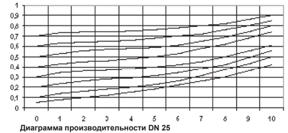
Диаграмма производительности DN 25
