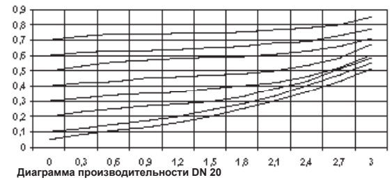
Диаграмма производительности DN 20
