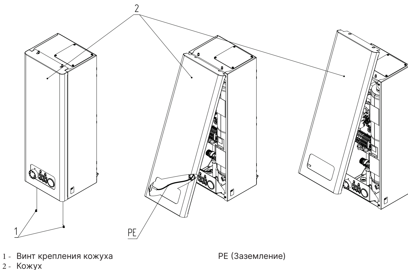
Рис.11 Демонтаж кожуха
