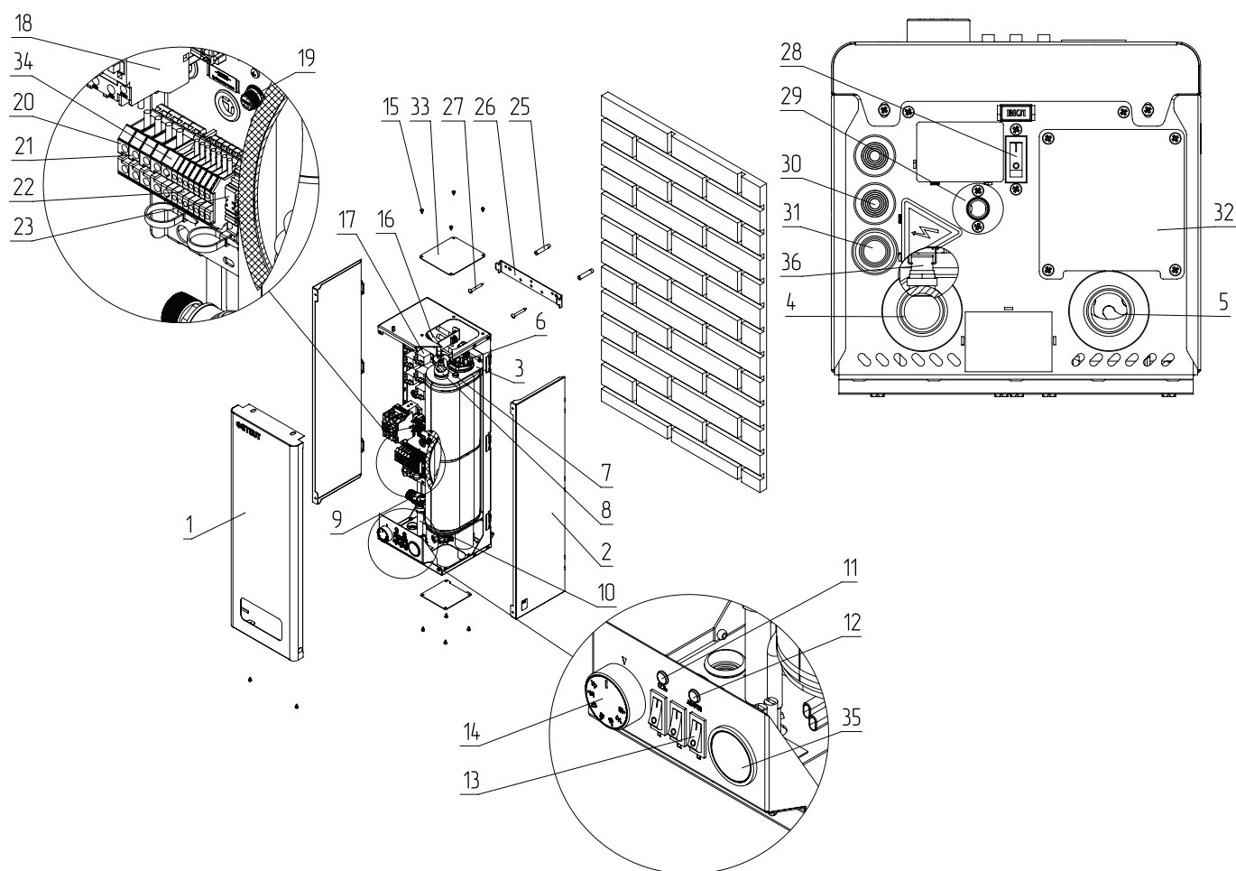
Рис.1 Устройство котла
