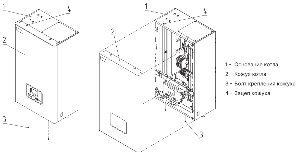
Рис.11 Снятие кожуха
