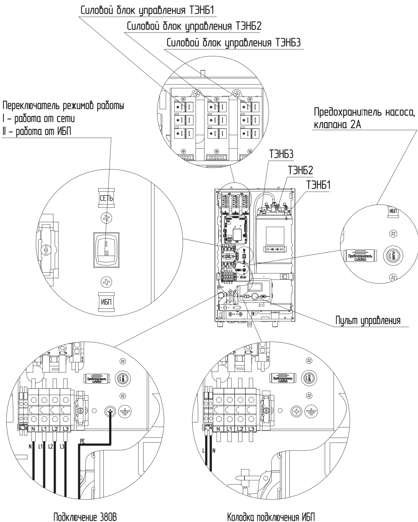
Рис.5 Схема подключения котла электрического STOUT STATUS 12-27 кВт
