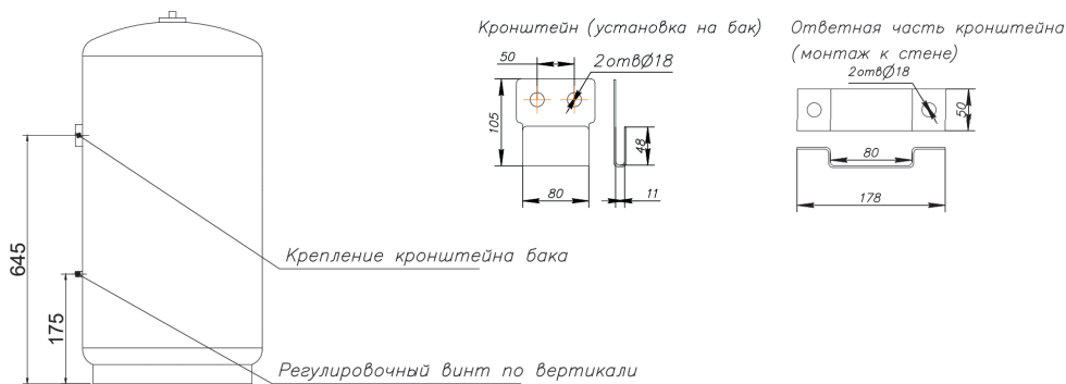
Рис. 4. Конструкция кронштейна настенного крепления
