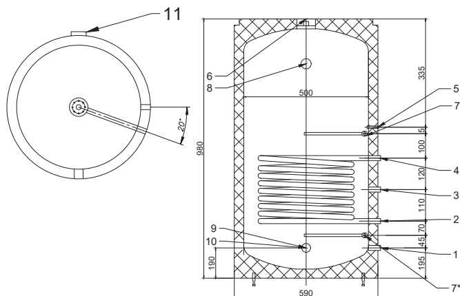
Рис. 1. Размеры SWH-2210-R/L00150
