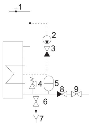
Рис. 5. Гидравлическая схема подключения бойлера
