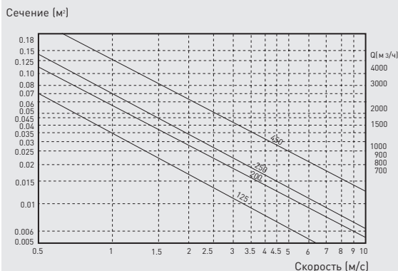
Зависимость расхода воздуха от скорости
