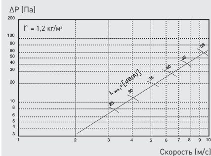
Потери давления и уровень шума (дБ(A))
