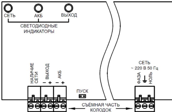
Рисунок 2 - Общий вид платы
