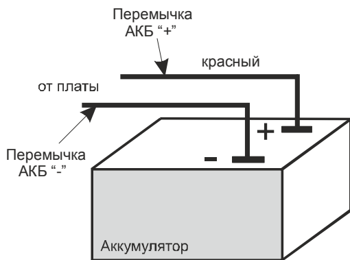
Рисунок 5. Подключение АКБ
