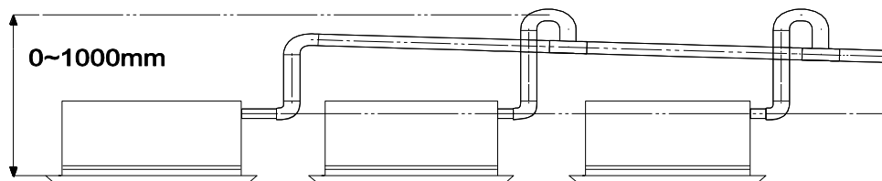
Сливные трубки, соединенные Т-муфтами
