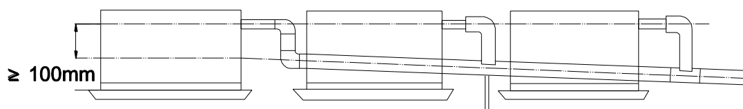
Сливные трубки, соединенные Т-муфтами
