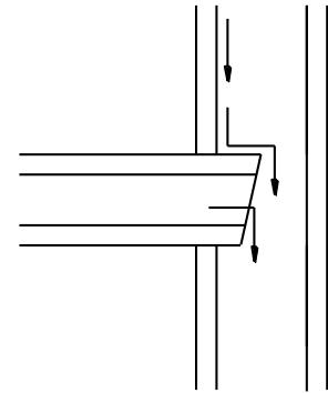
Скошенное устье горизонтальной трубки
