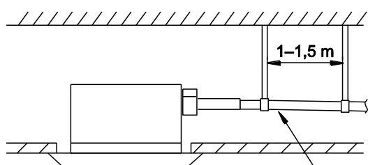
Правильно (наклон мин. 1/100)
