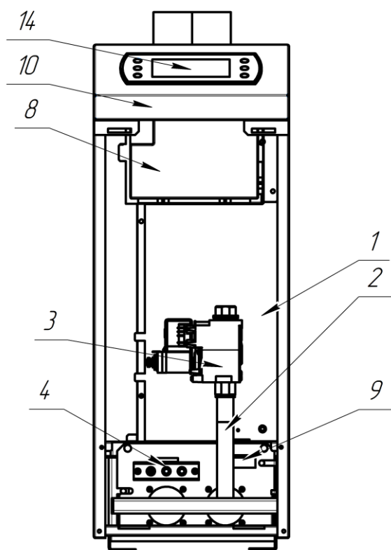
Рисунок 1 – Конструкция котла КОВ-СК(В)Ce
