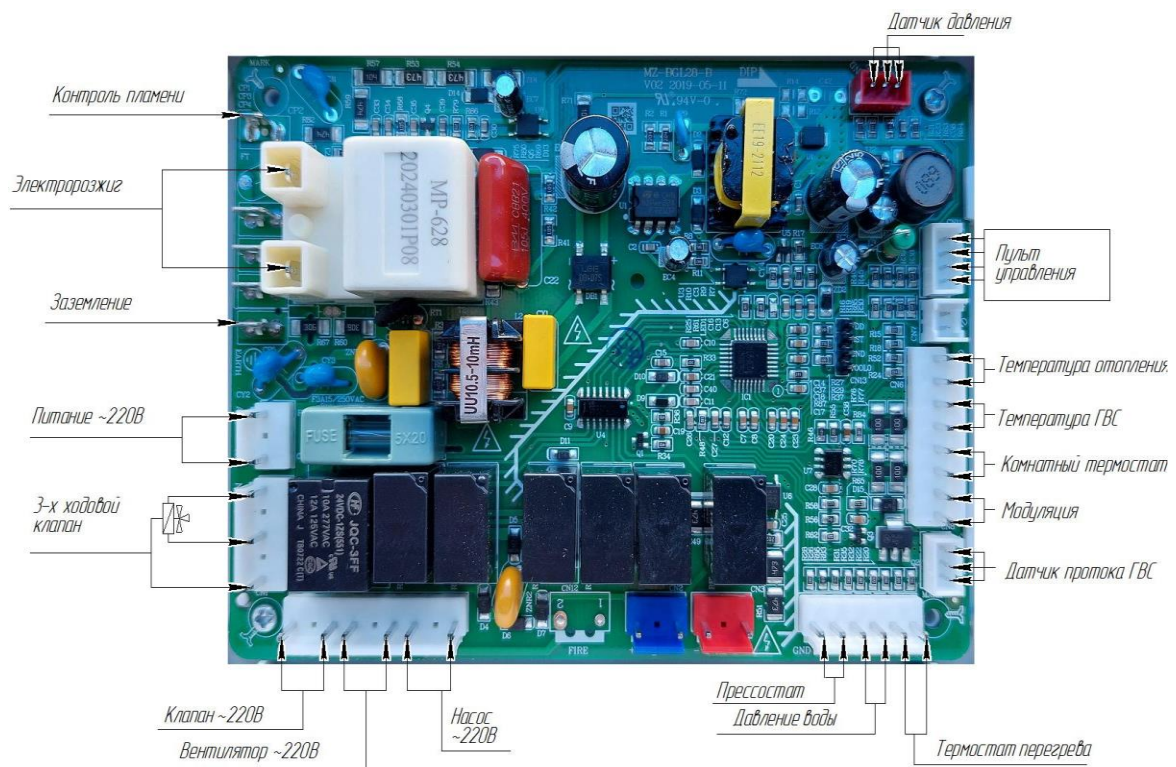
Рисунок 2 – Схема электрических подключений котла КОВ -___ СК(В)Се
