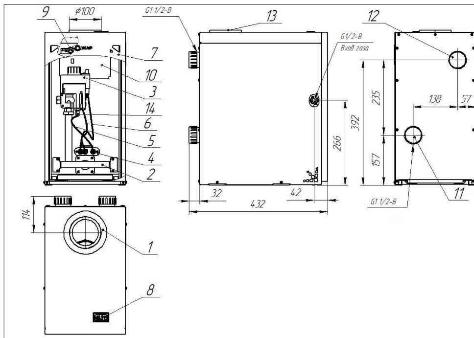
Рисунок 2 – Котел КОВ-СВПС «Сигнал»
