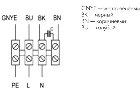
Схема 3
