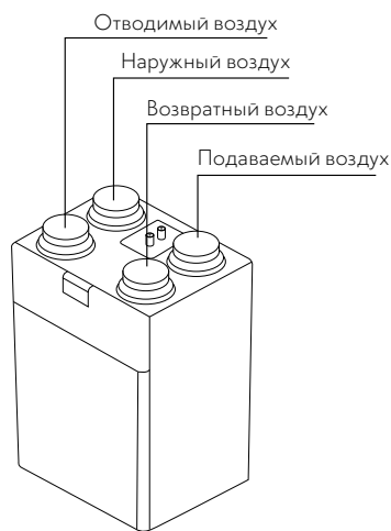
Установка левого типа (настраивается на месте монтажа)
