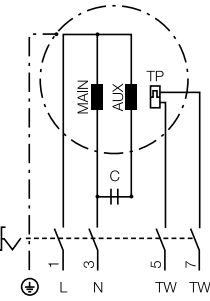
Схема 1
