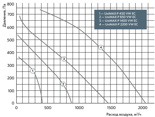
С водяным нагревом (VW)
