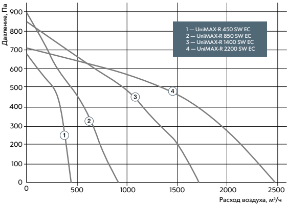
С водяным нагревом (SW)
