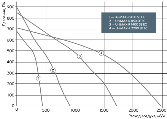
С электрическим нагревом (SE)
