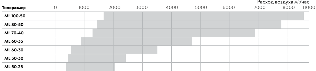
Номограмма для определения расхода воздуха серии ML
