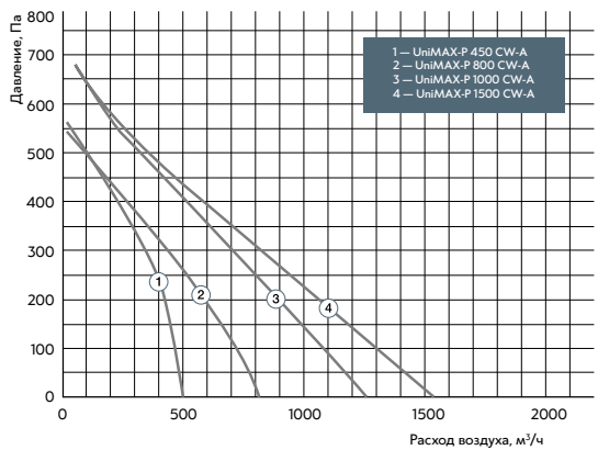
С водяным нагревом (CW)
