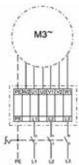
Схема 2
