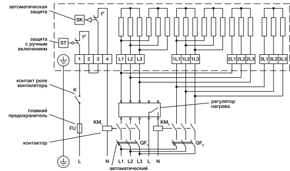
36, 45 кВт
