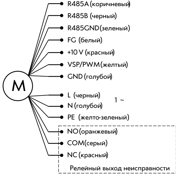
Схема 1
