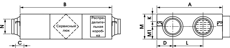
PVS 650–1100
