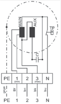
Схема 2
