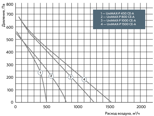
С электрическим нагревом (CE)
