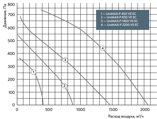
С электрическим нагревом (VE)
