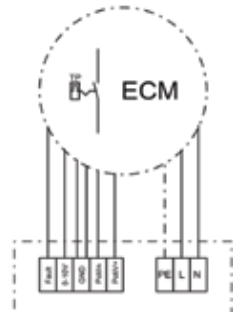
Схема 1
