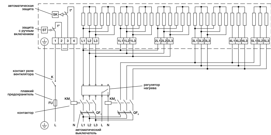
75 кВт
