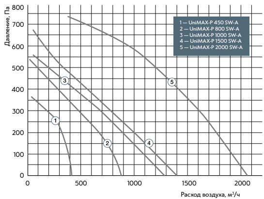
С водяным нагревом (SW)
