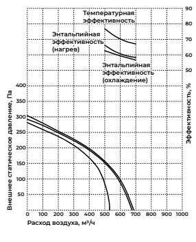
PVS-650
