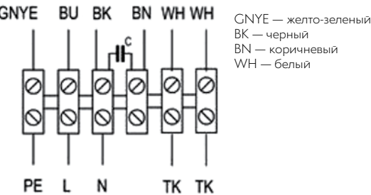
Схема 4
