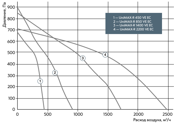
С электрическим нагревом (VE)
