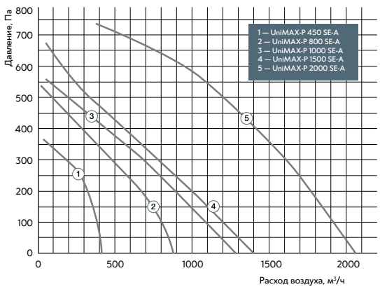
С электрическим нагревом (SE)
