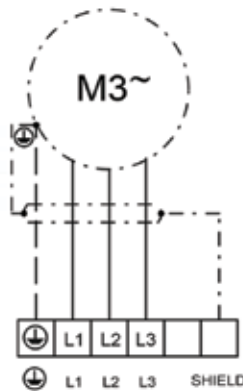
Схема 3
