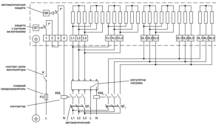
60 кВт
