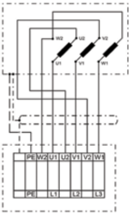
Схема 2
