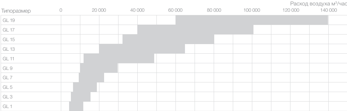
Номограмма для определения расхода воздуха серии GL
