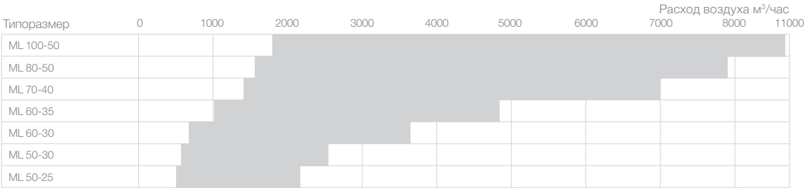
Номограмма для определения расхода воздуха серии ML
