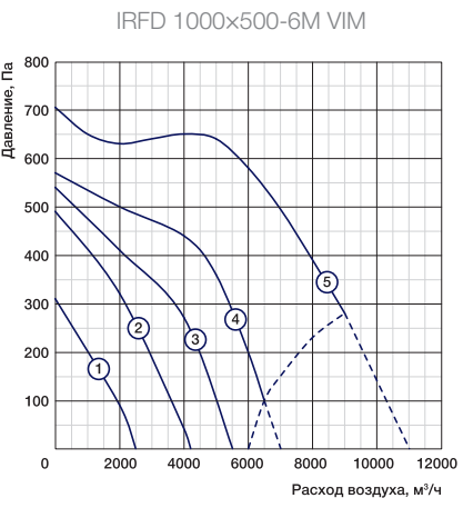
Частные характеристики 80-105-130-160-230 В
