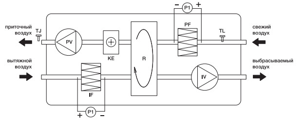
UniMAX-R 450/850/1400/2200 SW-A
