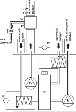
UniMAX-R 450 VW-A
