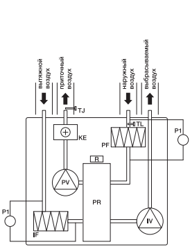
UniMAX-R 450 VE-A
