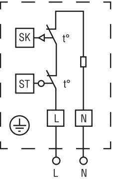
Схема 1 (230 В, 1 фаза)
