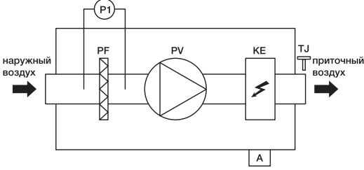
Принципиальная схема установок
