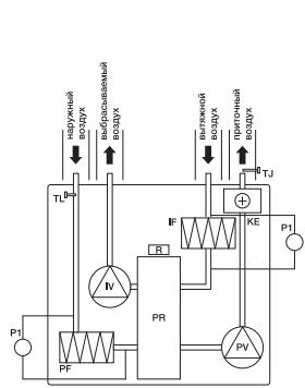
UniMAX-R 850/1400/2200 VE-A
