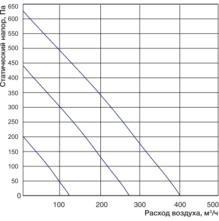
NOVA-600 EC
