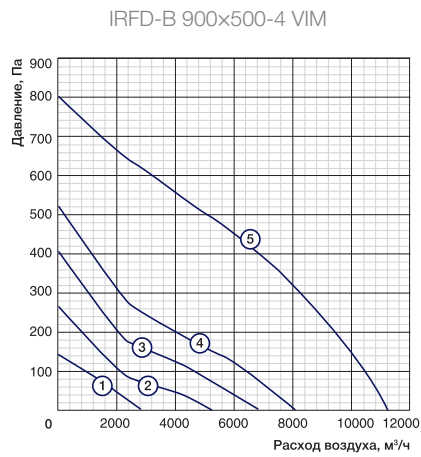
Частные характеристики 80-105-130-160-230 В
