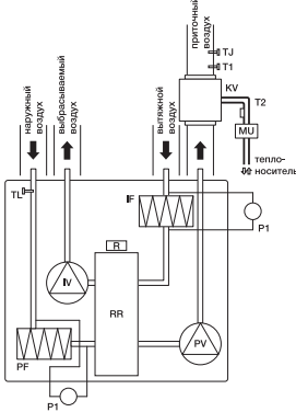
UniMAX-R 850/1400/2200 VW-A
