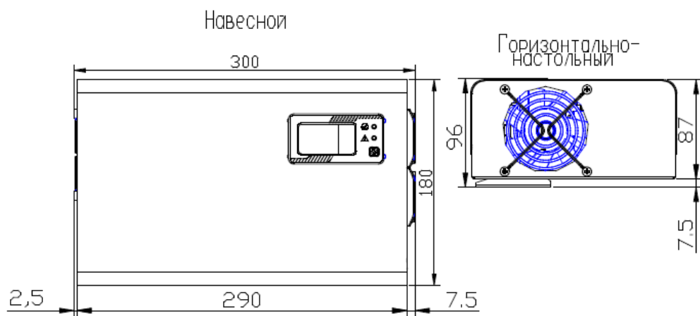
б) ИнСтаб IS1000; ИнСтаб IS1500
