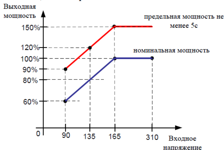
Рисунок 4 – Зависимость выходной мощности от входного напряжения
