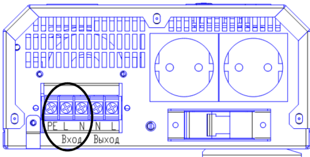
Рисунок 3.2 – Стабилизатор ИнСтаб IS2500 и ИнСтаб IS3500.
