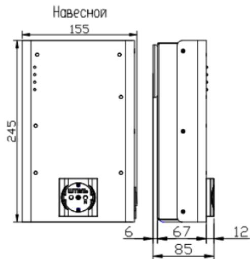
а) ИнСтаб IS350, ИнСтаб IS550
