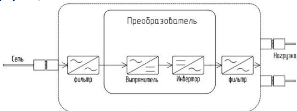
Рисунок 2 - Структурная схема принципа работы стабилизатора
