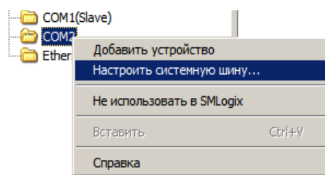
Рис. 51 –Настройка сети
