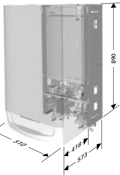
Isofloor et Isosplit montés
