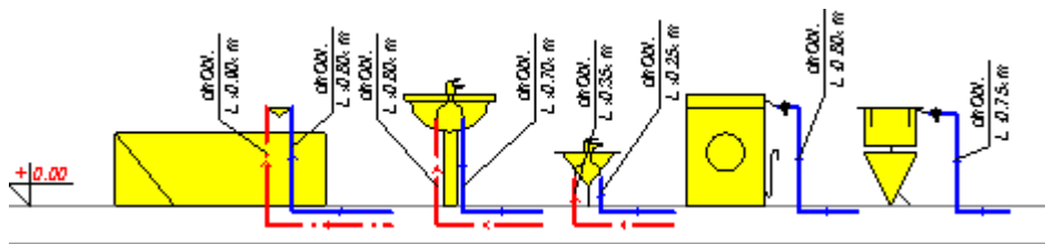
Элементы системы по схеме с распределительной разводкой в ванной
