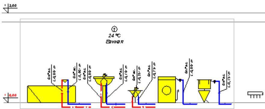
После вставки распределителя и растягивания его до четырех отводов
