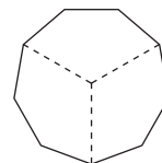
9-Kant-Profil 42 mm + 54 mm
