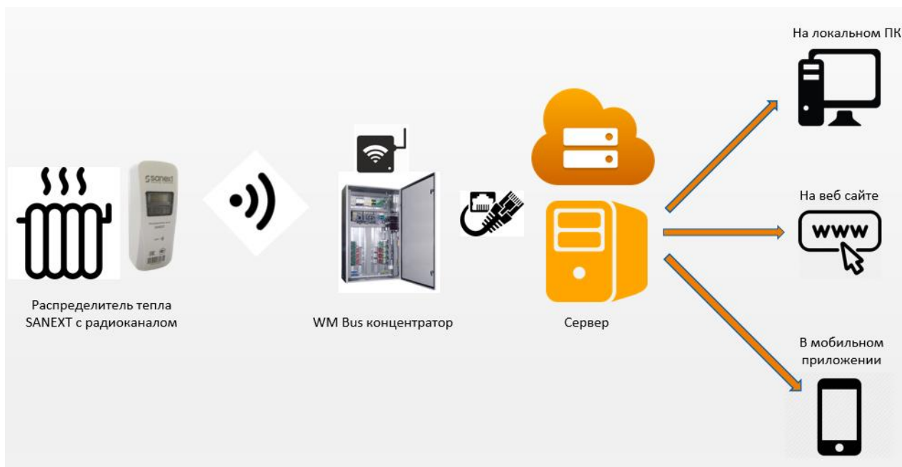
Рис. 2. Типовая схема чтения и передачи данных по радиоканалу Wireless Mbus
